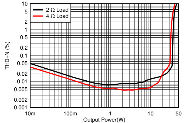
图 6-2. THD+N vs Power - 2 \Omega , 4 \Omega - 18 V
