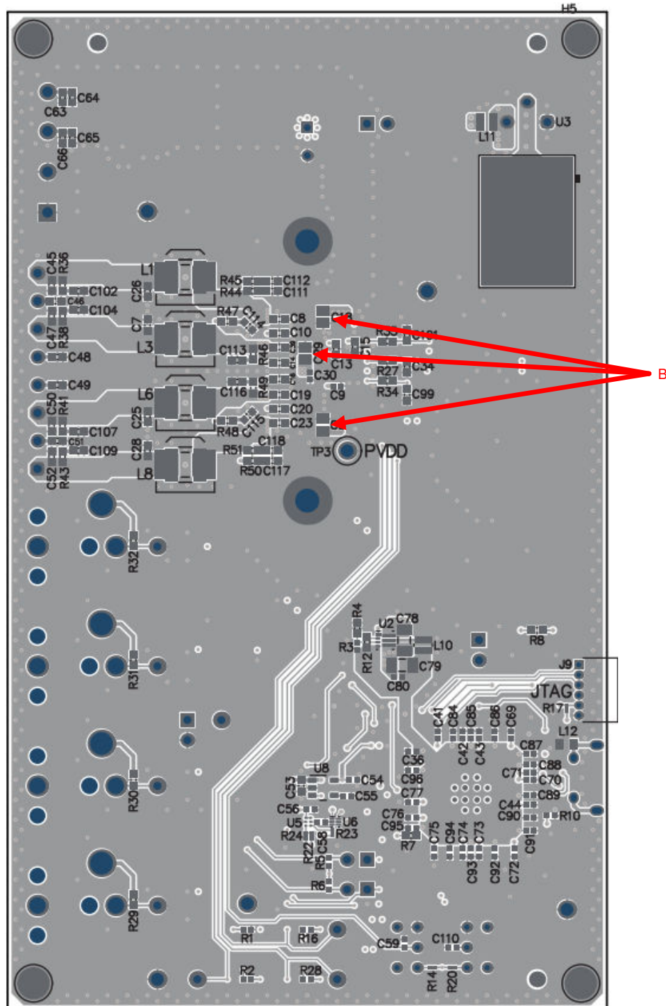
图 10-2. Layout Bottom Example
