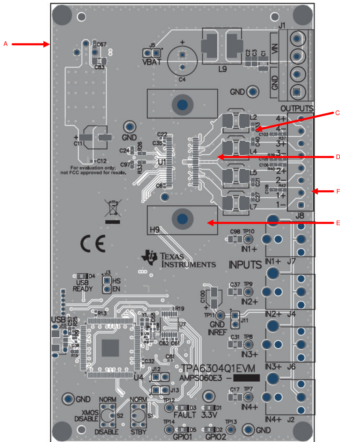
图 10-1. Layout Top Example
