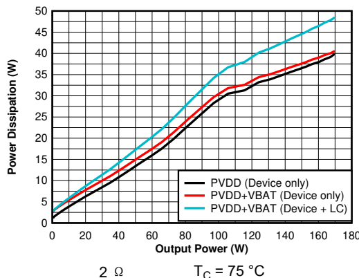
图 6-10. Power Dissipation vs Output Power - 2 Ω
