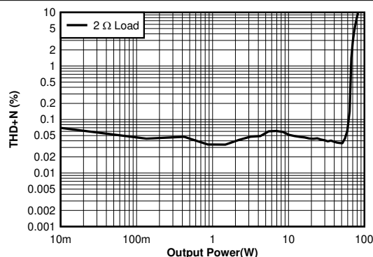
图 6-19. THD+N vs Power - PBTL, 2 Ω, 18 V
