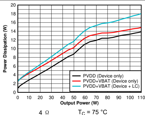
图 6-7. Power Dissipation vs Output Power - 4 Ω
