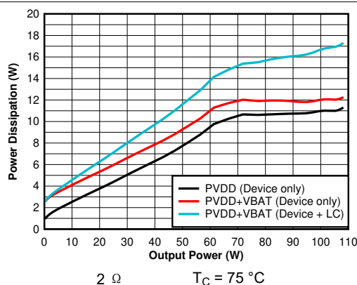
图 6-23. Power Dissipation vs Output Power - PBTL, 2 Ω
