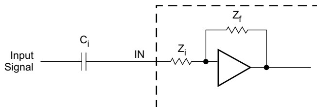
图 28. Input Impedance
