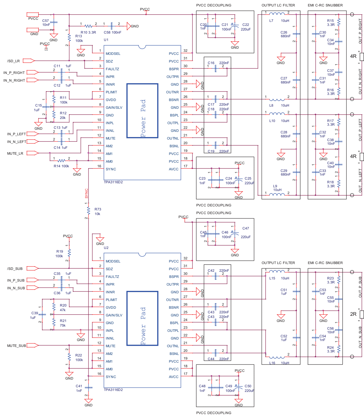
图 37. Schematic
