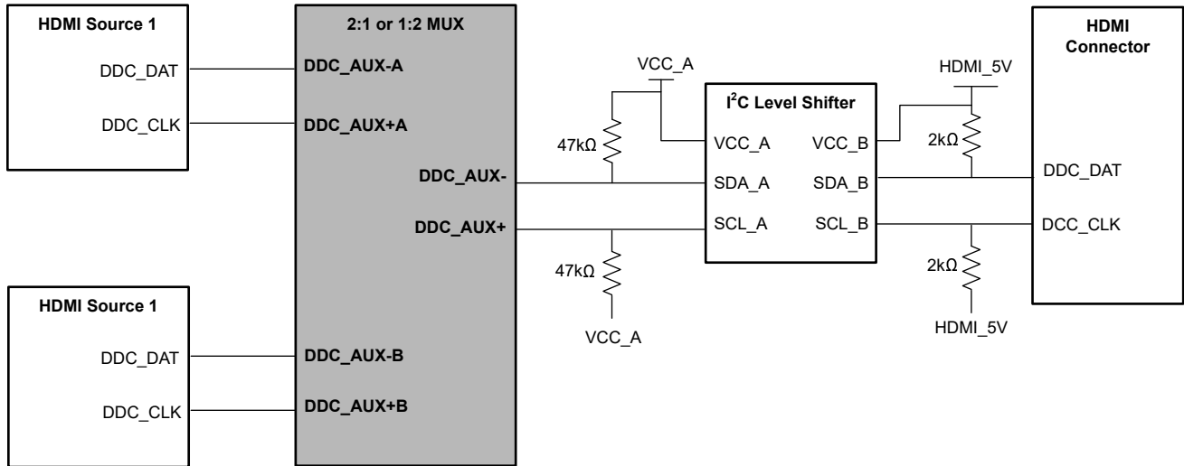
图 8-2. DDC 电平转换器源端侧示例
