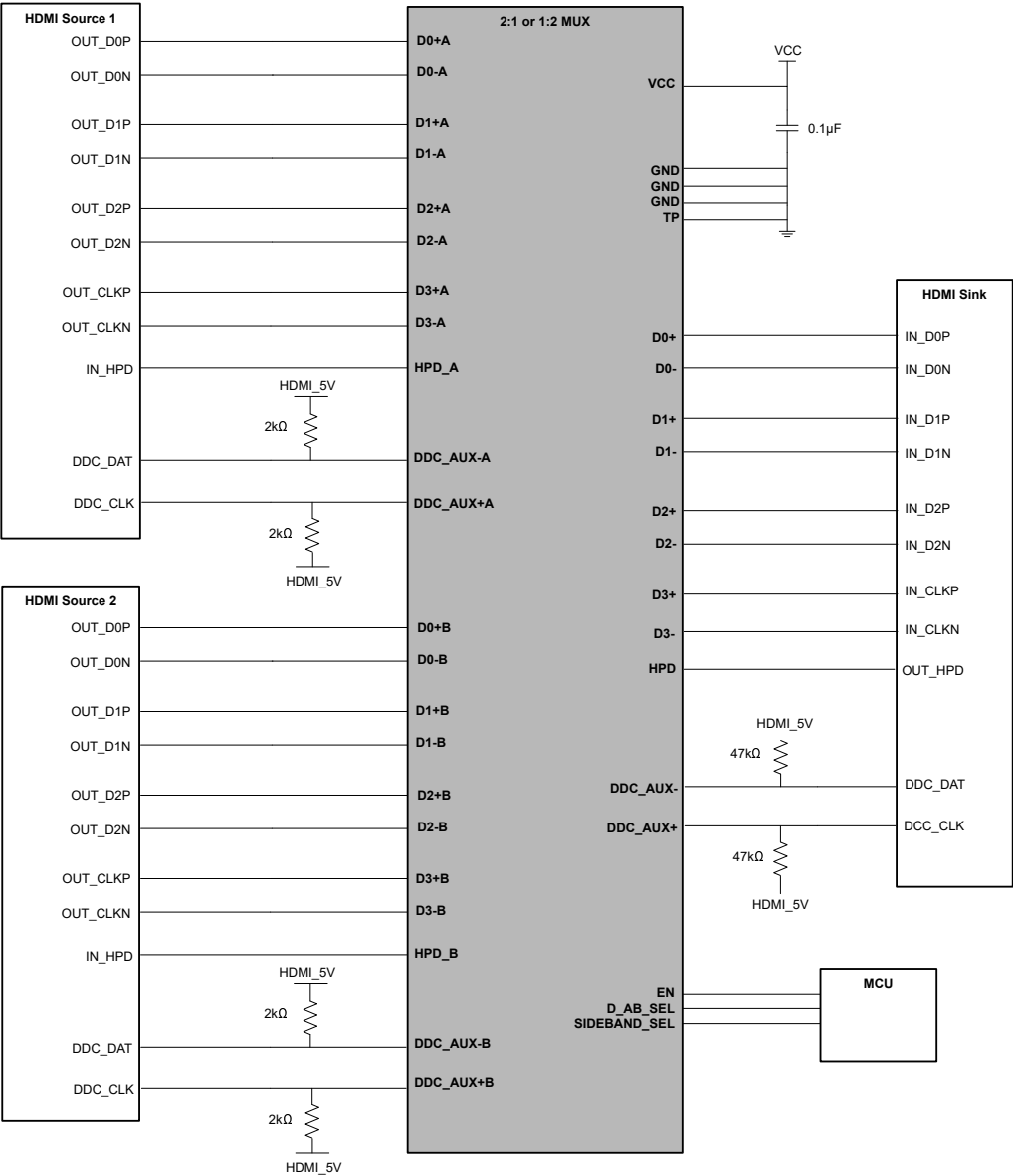
图 8-1. 选择两个 HDMI 端口之一 - 应用原理图
