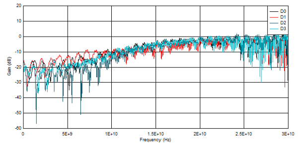
图 5-4. 选择端口 A 时的输出差分回波损耗
