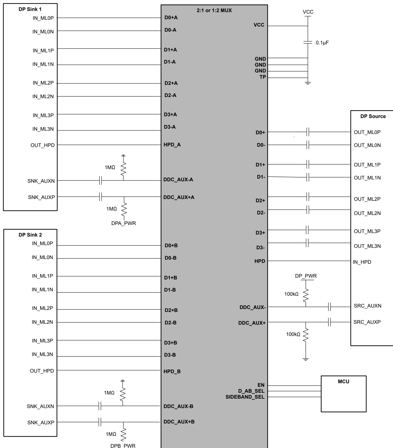
图 8-8. DisplayPort 1:2 开关
