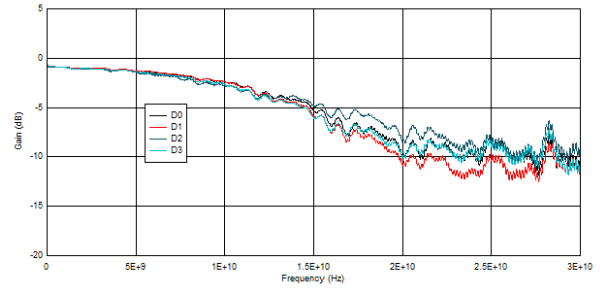
图 5-2. 端口 B 的差分插入损耗
