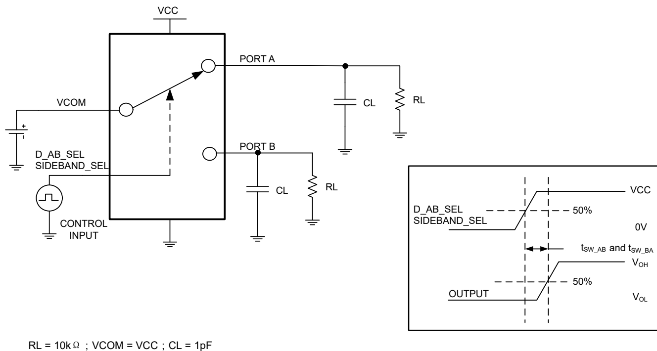
图 6-2. 通道间的切换时间 ( t_{SW\_AB} 和 t_{SW\_BA} )
