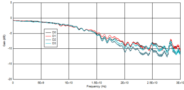
图 5-1. 端口 A 的差分插入损耗
