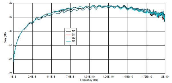
图 5-6. 端口 A 的关断状态隔离 (OISO)
