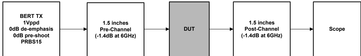
图 8-3. 测试设置
