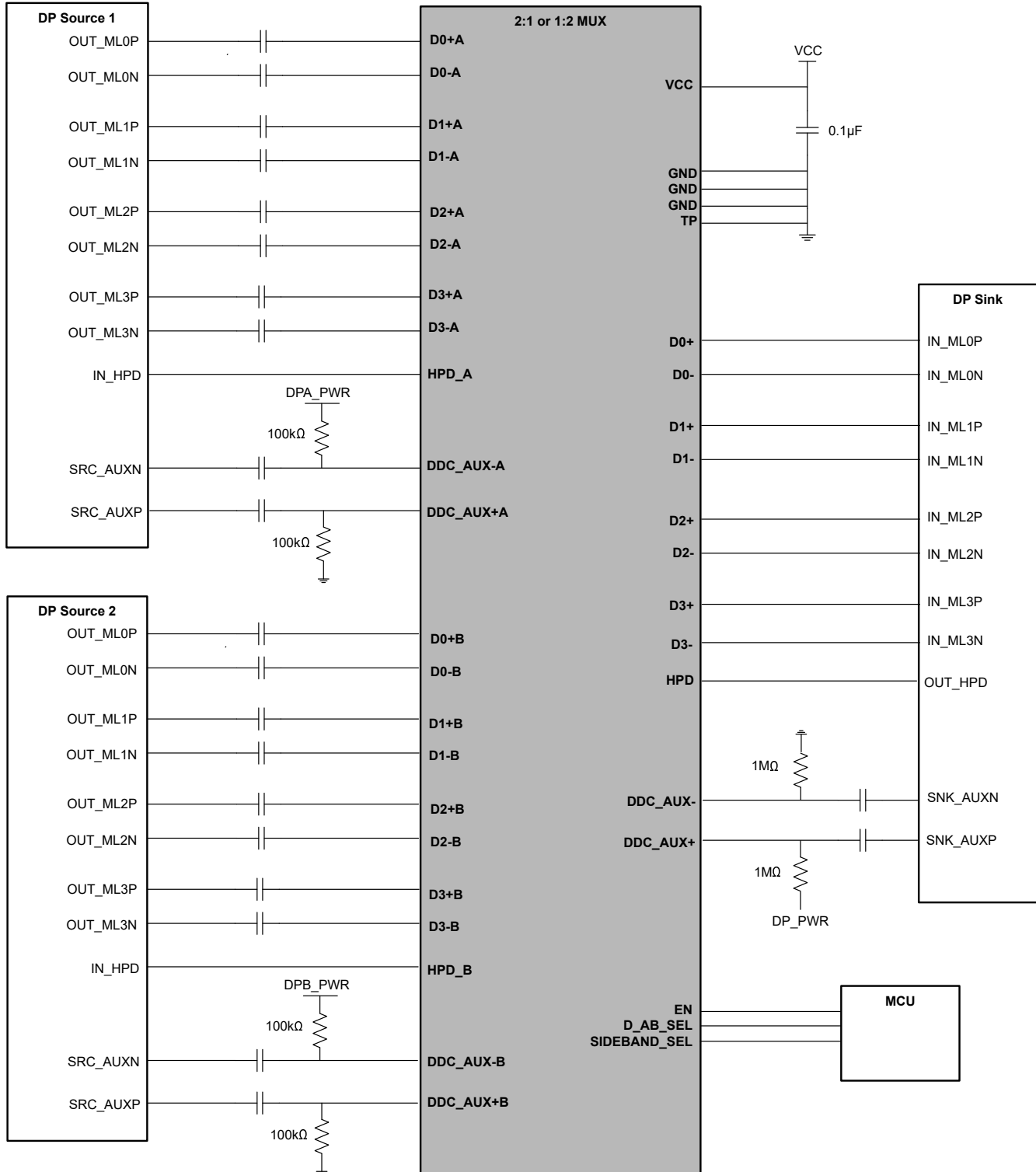
图 8-7. DisplayPort 2:1 开关
