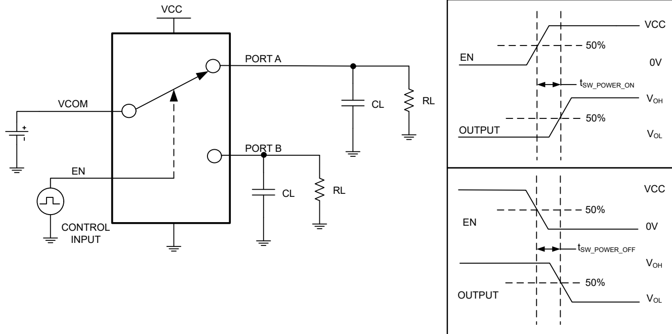
图 6-1. 开关导通时间 ( t_{SW\_POWER\_ON} 和 t_{SW\_POWER\_OFF} )
