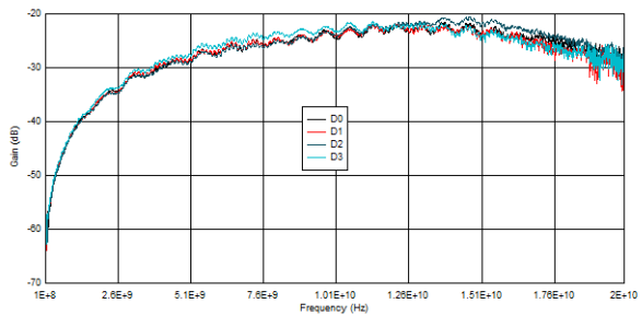
图 5-7. 端口 B 的关断状态隔离 (OISO)
