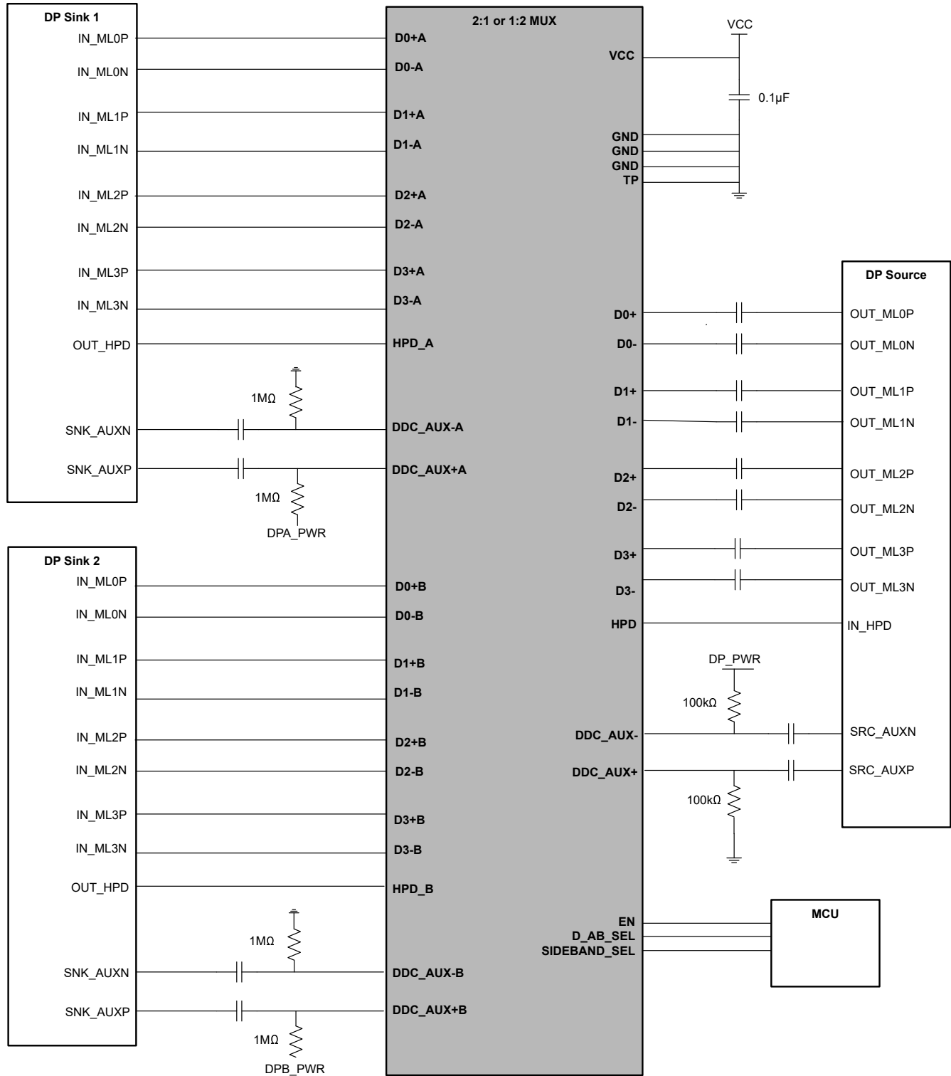
图 8-6. DisplayPort 1:2 开关
