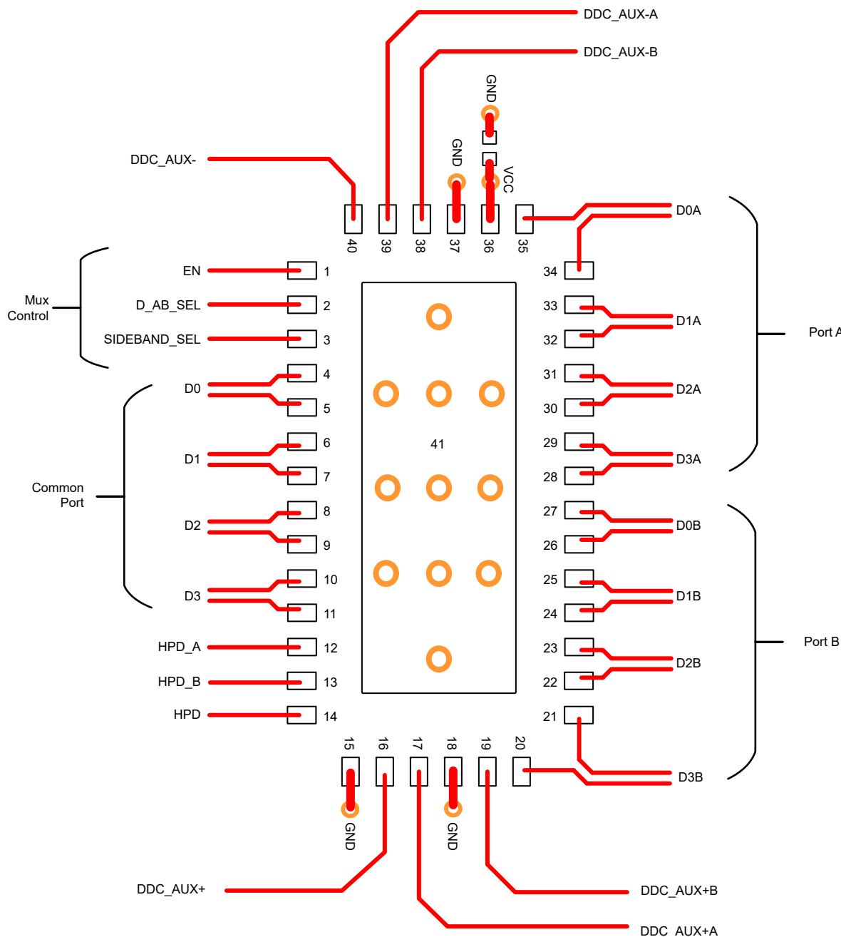
图 8-5. 布局示例
