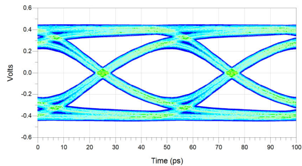
图 8-4. 眼图：20Gbps 端口 B，D0+ 到 D0-B（一次只测量一个通道）
