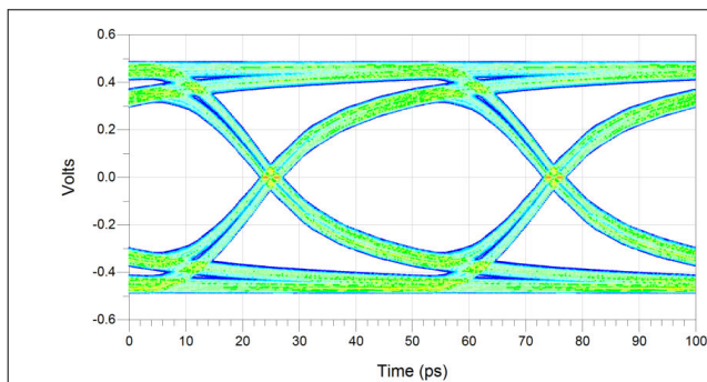
图 8-3. 眼图：20Gbps，无器件直通路径（一次只测量一个通道）
