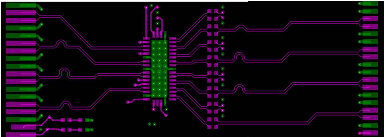
图 7-11. TMUXHS4412 Layout Example
