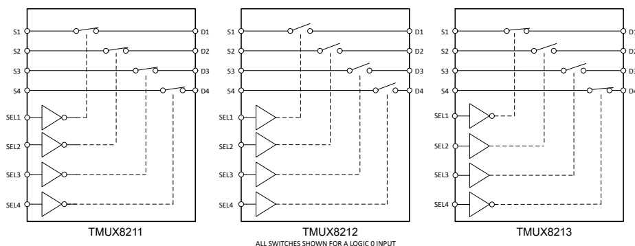
功能方框图
