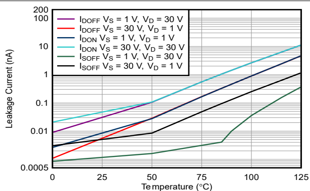
图 6-16. 漏电流与温度间的关系
