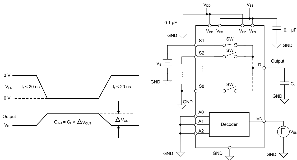
图 7-13. 电荷注入测量设置
