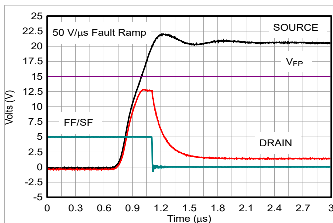
图 10-2. 正过压响应
