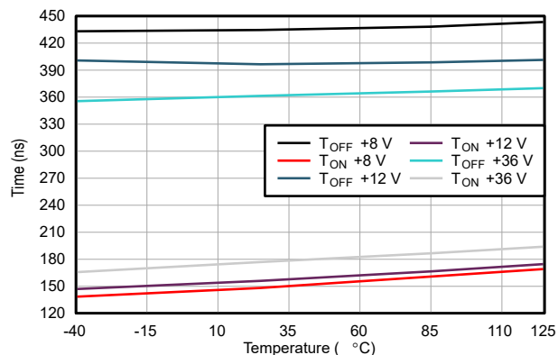
图 7-28. 转换时间与温度间的关系
