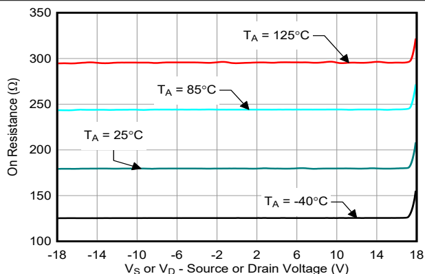
图 7-2. 导通电阻与源极或漏极电压之间的关系
