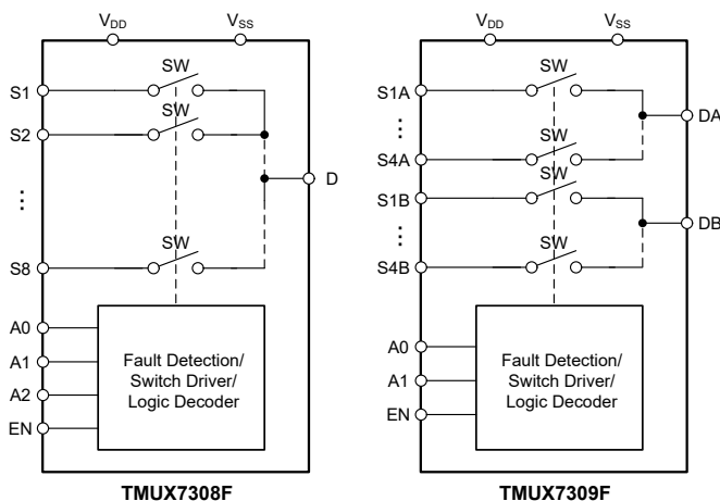
功能模块图
