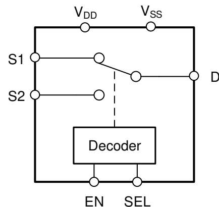
功能方框图
