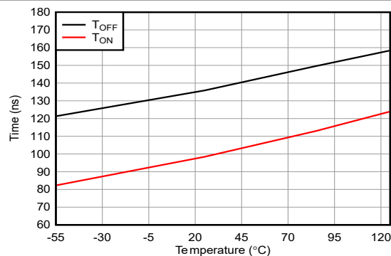
图 6-18. T_{ON} 和 T_{OFF} 与温度间的关系 V_{DD} = 15\text{ V}, V_{SS} = -15\text{ V}
