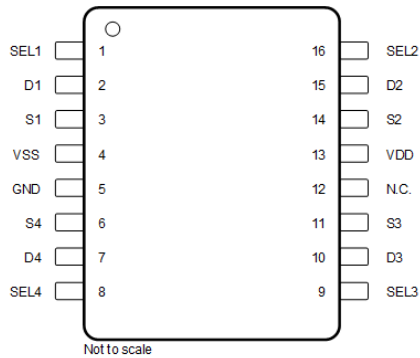
图 5-1. PW 封装，16 引脚 TSSOP ( 俯视图 )
