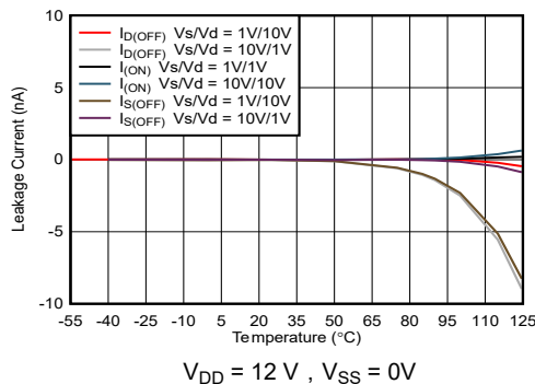
图 6-12. 漏电流与温度间的关系
