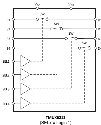
TMUX621x 功能方框图
