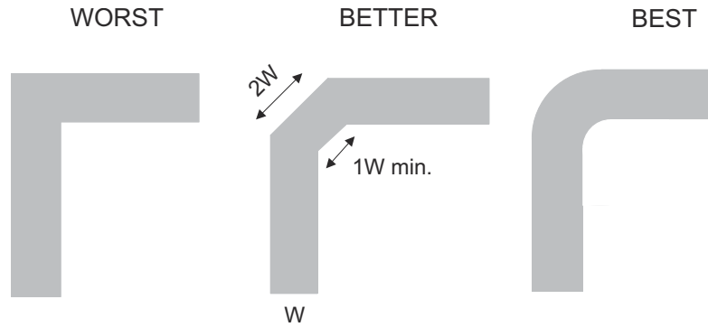
图 9-4. 布线示例
