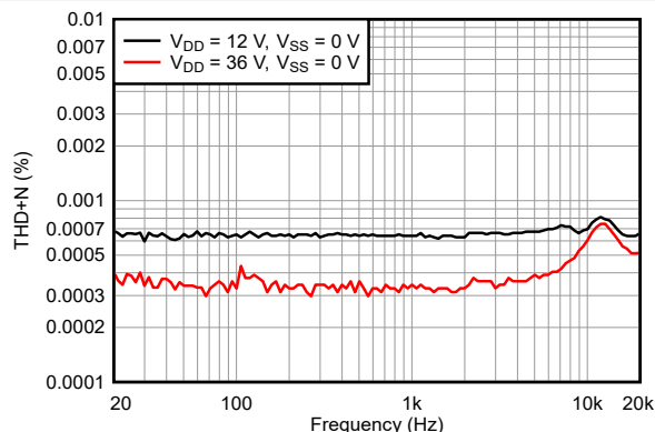
图 6-22. THD+N 与频率间的关系 (单电源)
