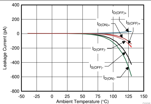
V_{DD} = 15\text{ V} , V_{SS} = -15\text{ V}
