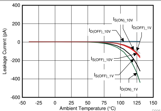
V_{DD} = 12\text{ V} , V_{SS} = 0\text{ V}
