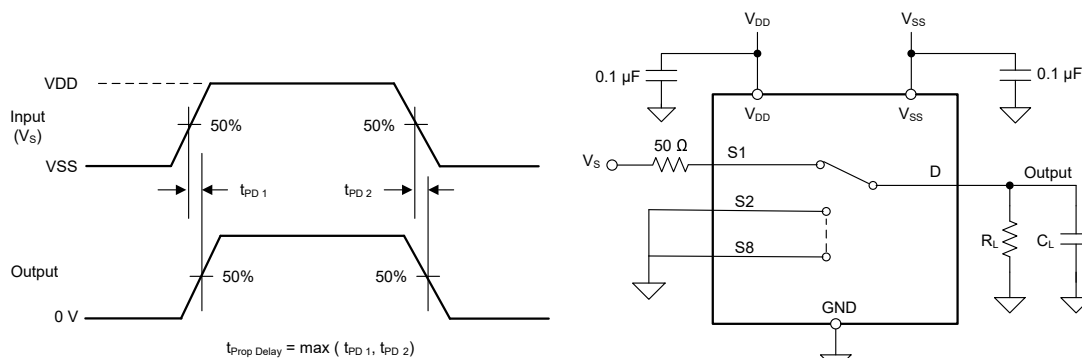
图 7-7. 传播延迟测量设置
