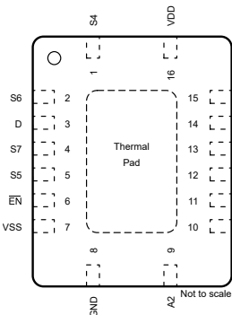
图 5-3. TMUX4051 BQB 封装，16 引脚 WQFN（顶视图）
