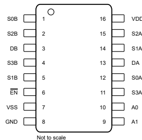
图 5-5. TMUX4052 DYY 封装, 16 引脚 SOT-23-THIN (顶视图)
