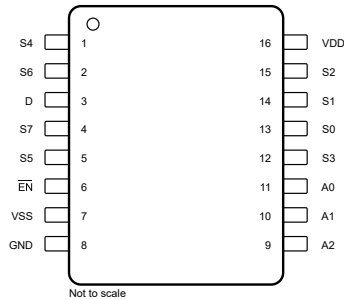
图 5-1. TMUX4051 PW 封装，16 引脚 TSSOP（顶视图）
