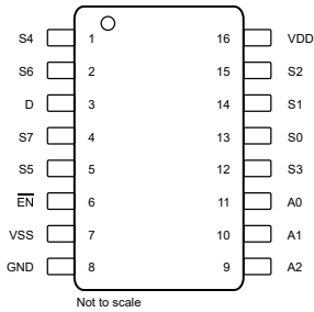
图 5-2. TMUX4051 DYY 封装，16 引脚 SOT-23-THIN（顶视图）
