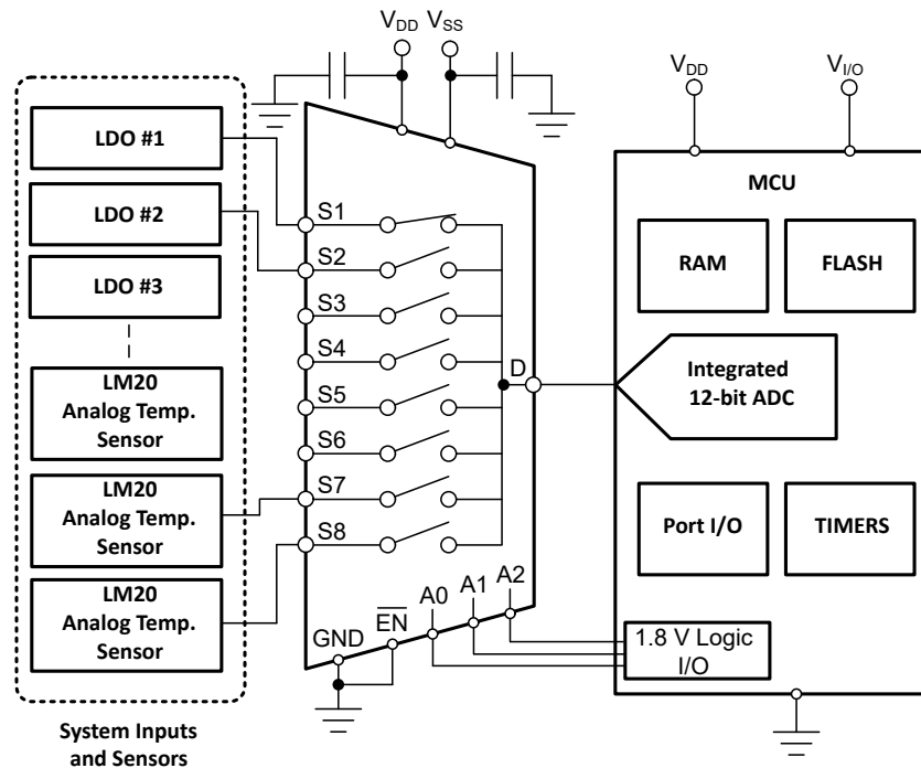
图 9-1. 使用 TMUX4051 将信号多路复用到集成 ADC
