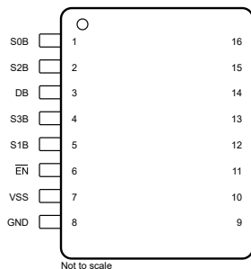
图 5-4. TMUX4052 PW 封装, 16 引脚 TSSOP (顶视图)
