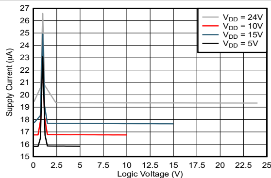
图 6-4. 电源电流与逻辑电压间的关系
