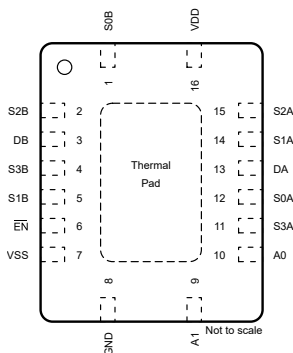
图 5-6. TMUX4052 BQB 封装, 16 引脚 WQFN (顶视图)
