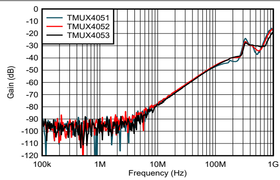
图 6-8. 关断隔离与频率间的关系
