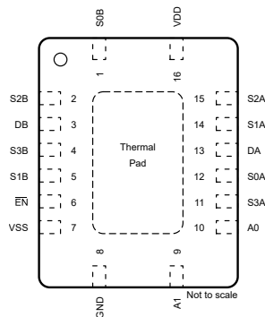
图 6-6. TMUX4052-Q1 BQB 封装，16 引脚 WQFN (顶视图)
