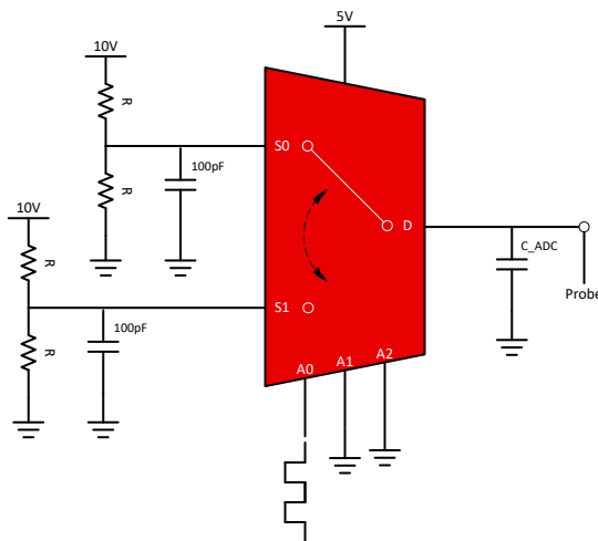
图 8-1. 测试电路设置
