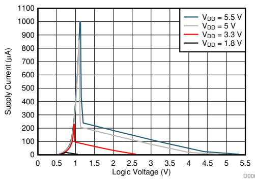
图 6-5. 电源电流与逻辑电压间的关系
