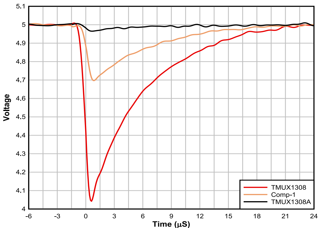
图 8-2. TMUX1308A 与竞争器件漏极稳定时间的比较
