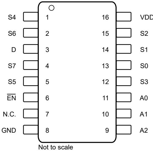
图 5-2. TMUX1308A : DYY 封装，16 引脚 SOT-23-THIN (顶视图)
