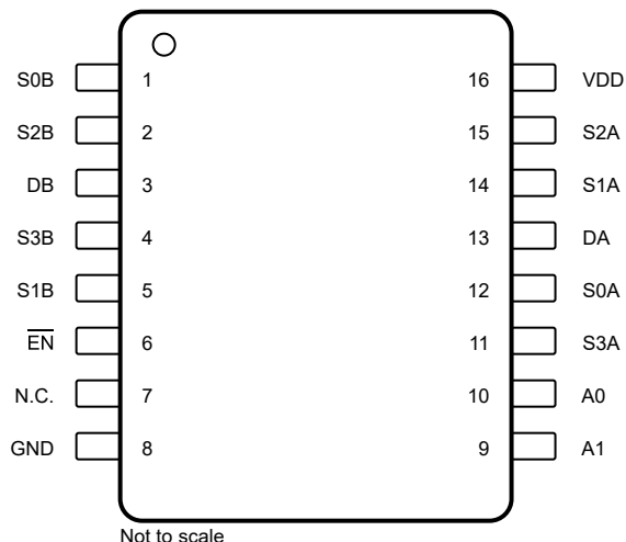
图 5-4. TMUX1309A : PW 封装 , 16 引脚 TSSOP ( 顶视图 )
