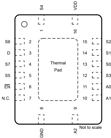
图 5-3. TMUX1308A : BQB 封装，16 引脚 WQFN (顶视图)
