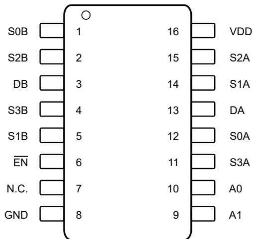
图 5-5. TMUX1309A : DYY 封装 , 16 引脚 SOT-23- THIN ( 顶视图 )
