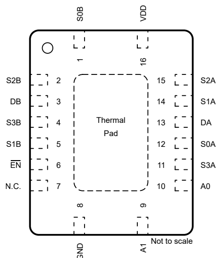
图 5-6. TMUX1309A : BQB 封装 , 16 引脚 WQFN ( 顶视图 )
