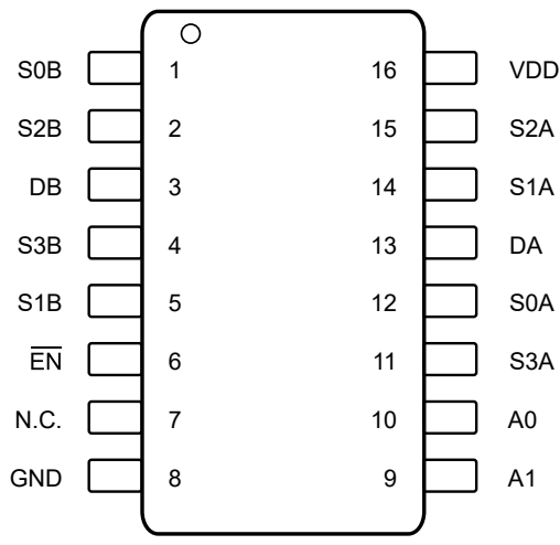
图 6-5. TMUX1309-Q1: DYY Package, 16-Pin SOT-23-THIN (Top View)
