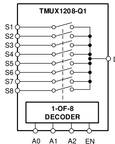
TMUX1208-Q1 方框图
