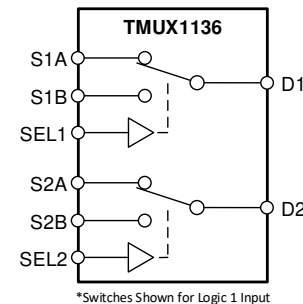
方框图
