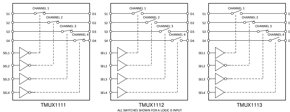
TMUX111x 方框图
