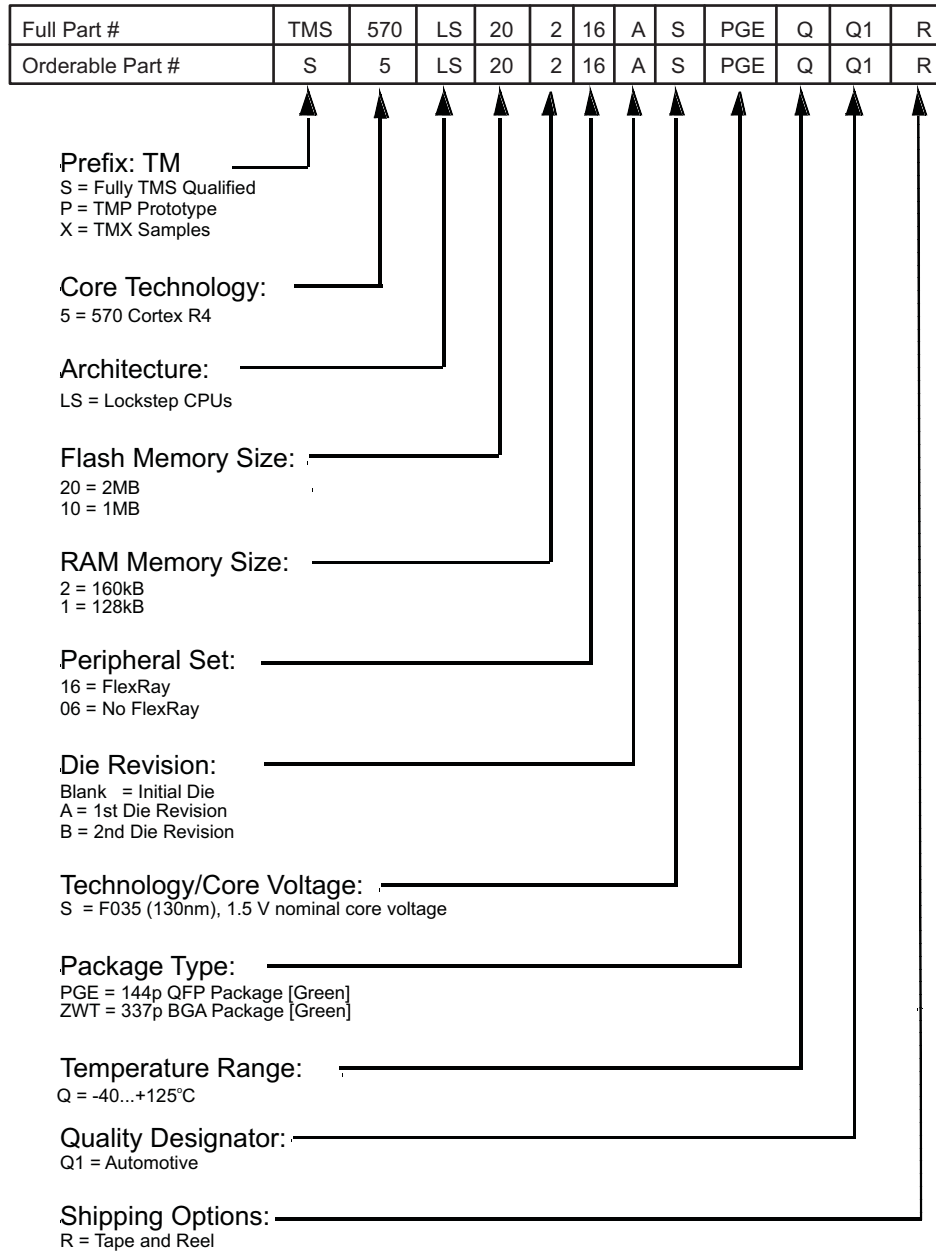
图 2-9. 器件编号惯例(A)
