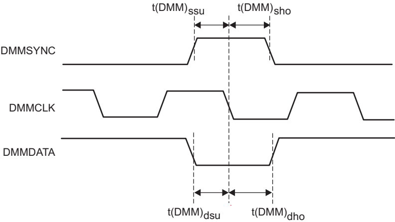
图 7-25. DMMDATA 时序
