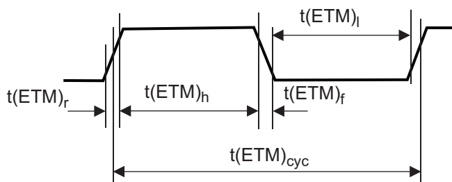
图 7-19. ETMTRACECLK 时序
