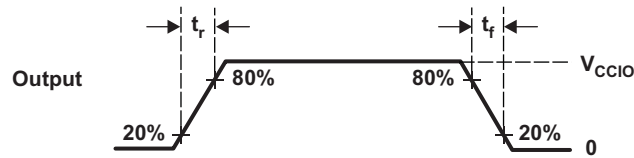
图 7-7. CMOS - 级输出
