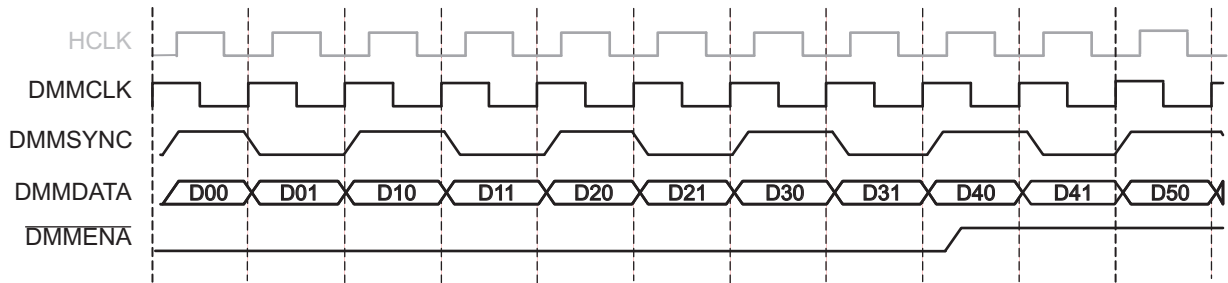
图 7-26. DMMENA 时序
