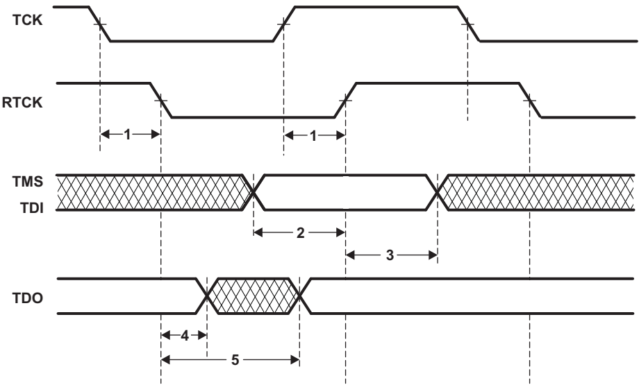
图 7-6. JTAG 的时序
