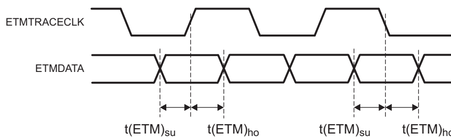
图 7-20. ETMDATA 时序
