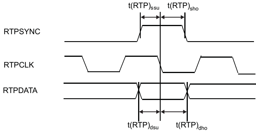
图 7-22. RTPDATA 时序
