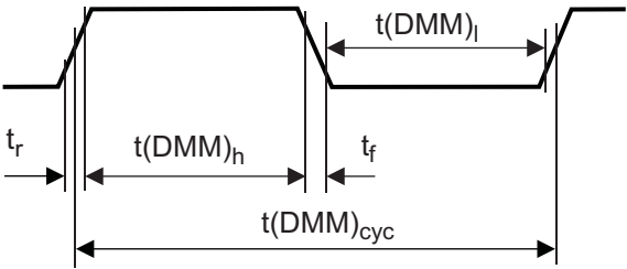
图 7-24. DMMCLK 时序
