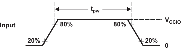
图 7-8. CMOS - 级输入
