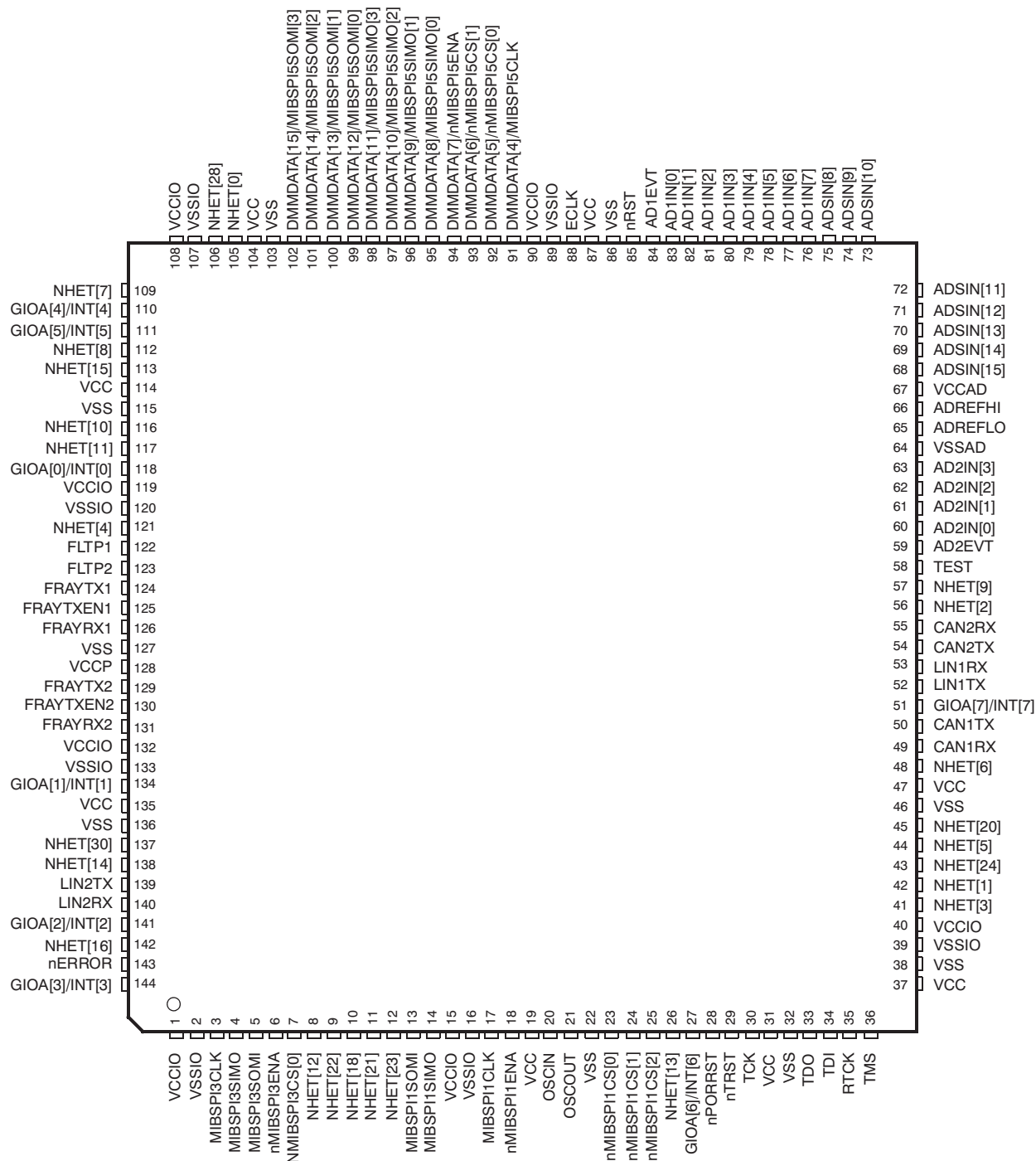
图 2-4. PGE 引脚分配 (144 引脚) [顶视图]
