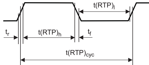
图 7-21. RTPCLK 时序
