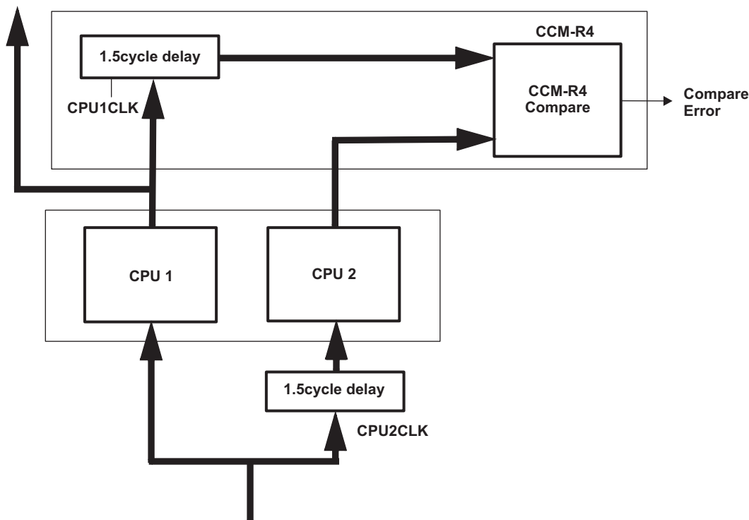
图 4-2. 双内核执行
