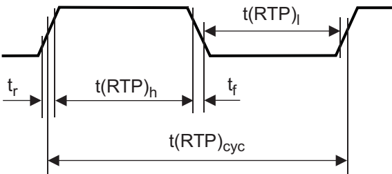
图 7-21. RTPCLK 时序
