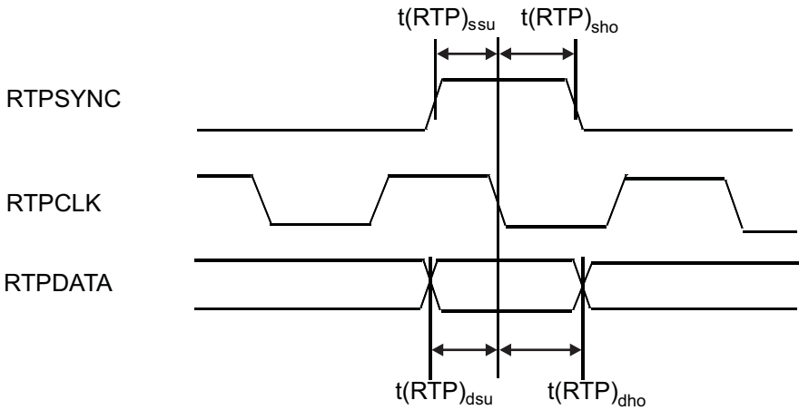
图 7-22. RTPDATA 时序
