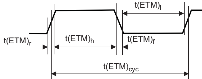
图 7-19. ETMTRACECLK 时序
