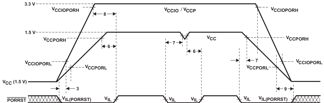
图 7-5. PORRST 时序图
