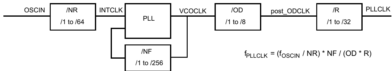
图 5-6. PLL Block Diagram
