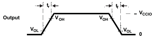
图 6-2. CMOS-Level Outputs
