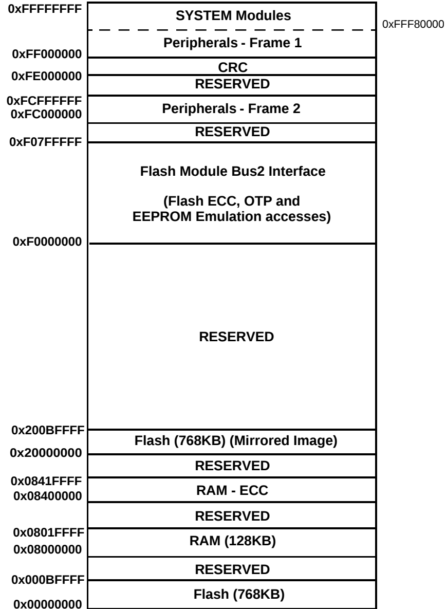
图 5-9. Memory Map
