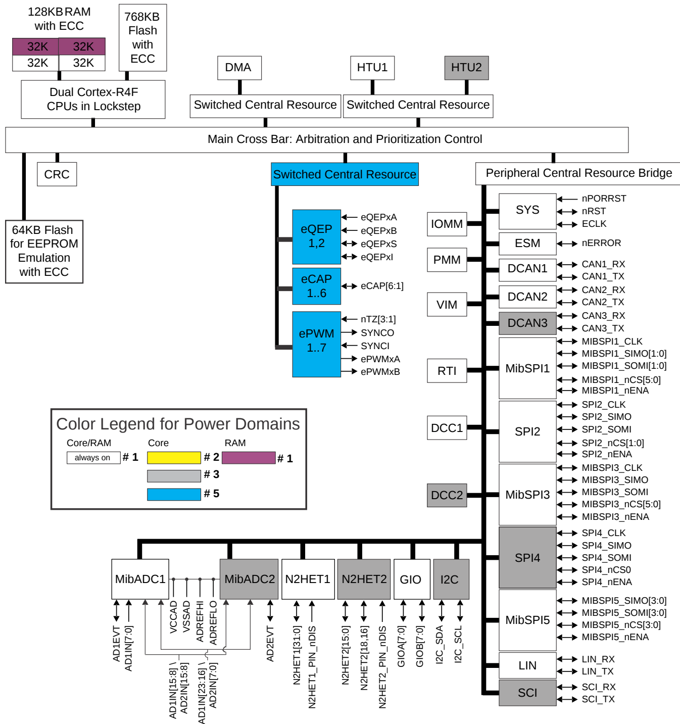
图 1-1. 功能框图
