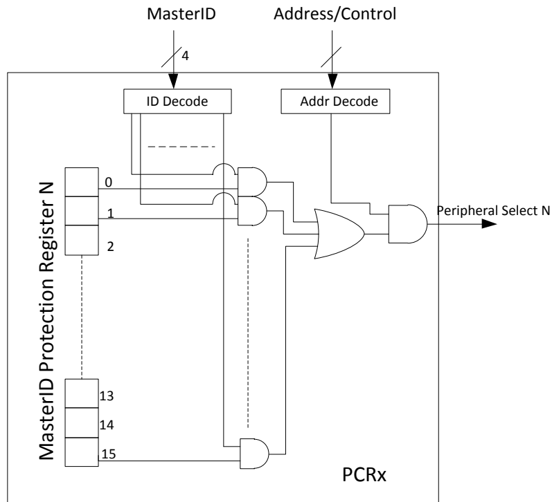
图 7-10. PCR MasterID Filtering
