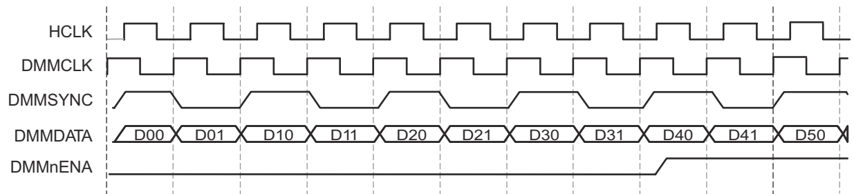
图 7-37. DMMnENA Timing
