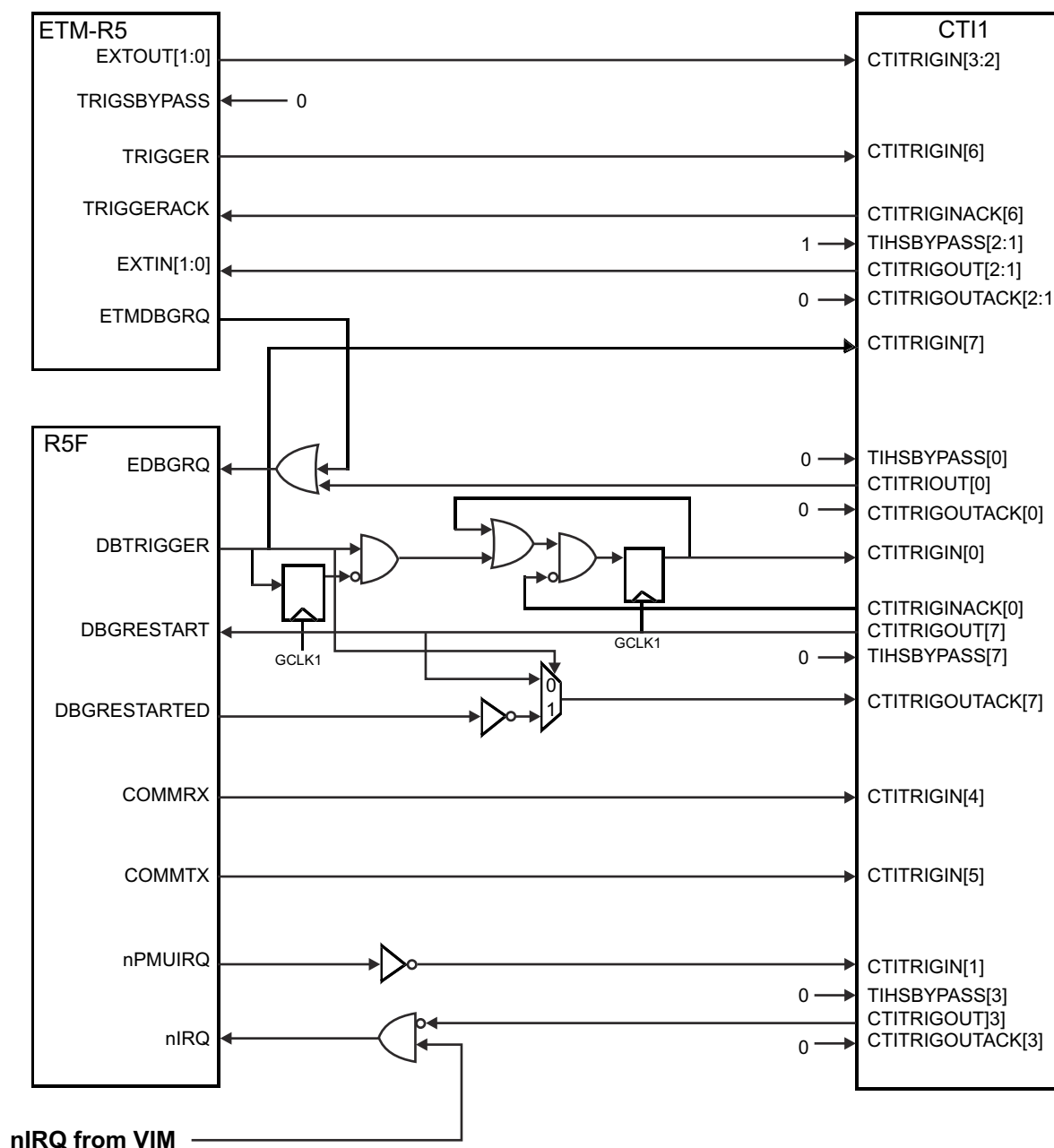
图 7-25. CTI1 Mapping
