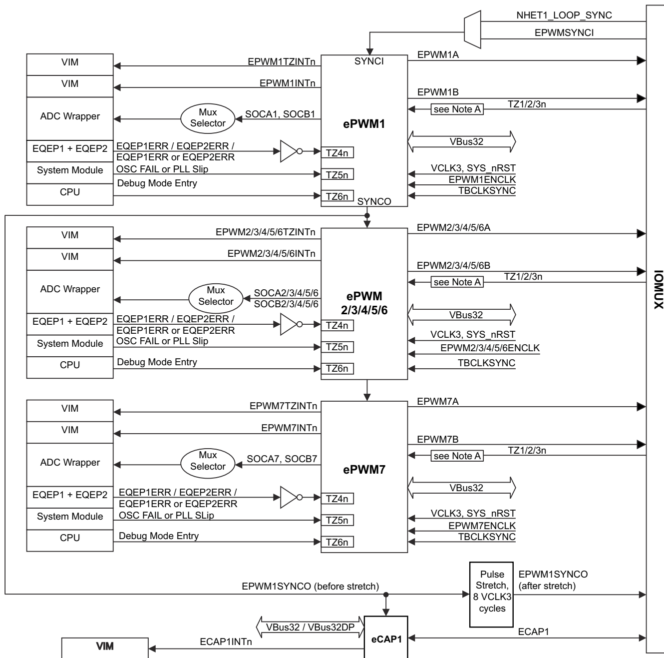
图 8-1. ePWMx Module Interconnections
