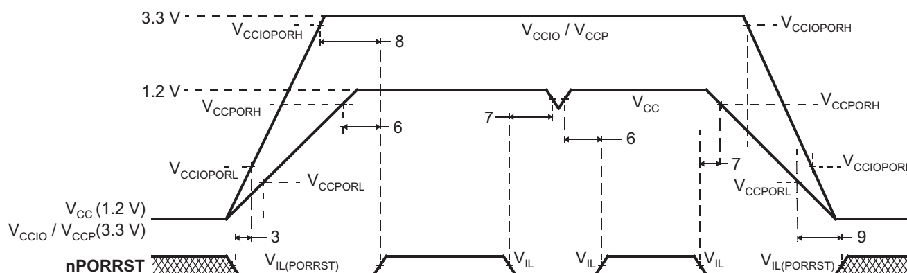
图 5-1. nPORRST 时序图
