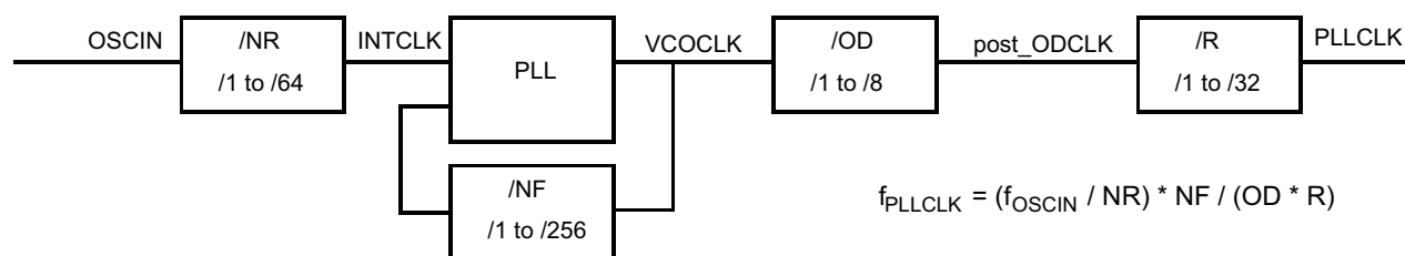
图 5-6. PLL 方框图
