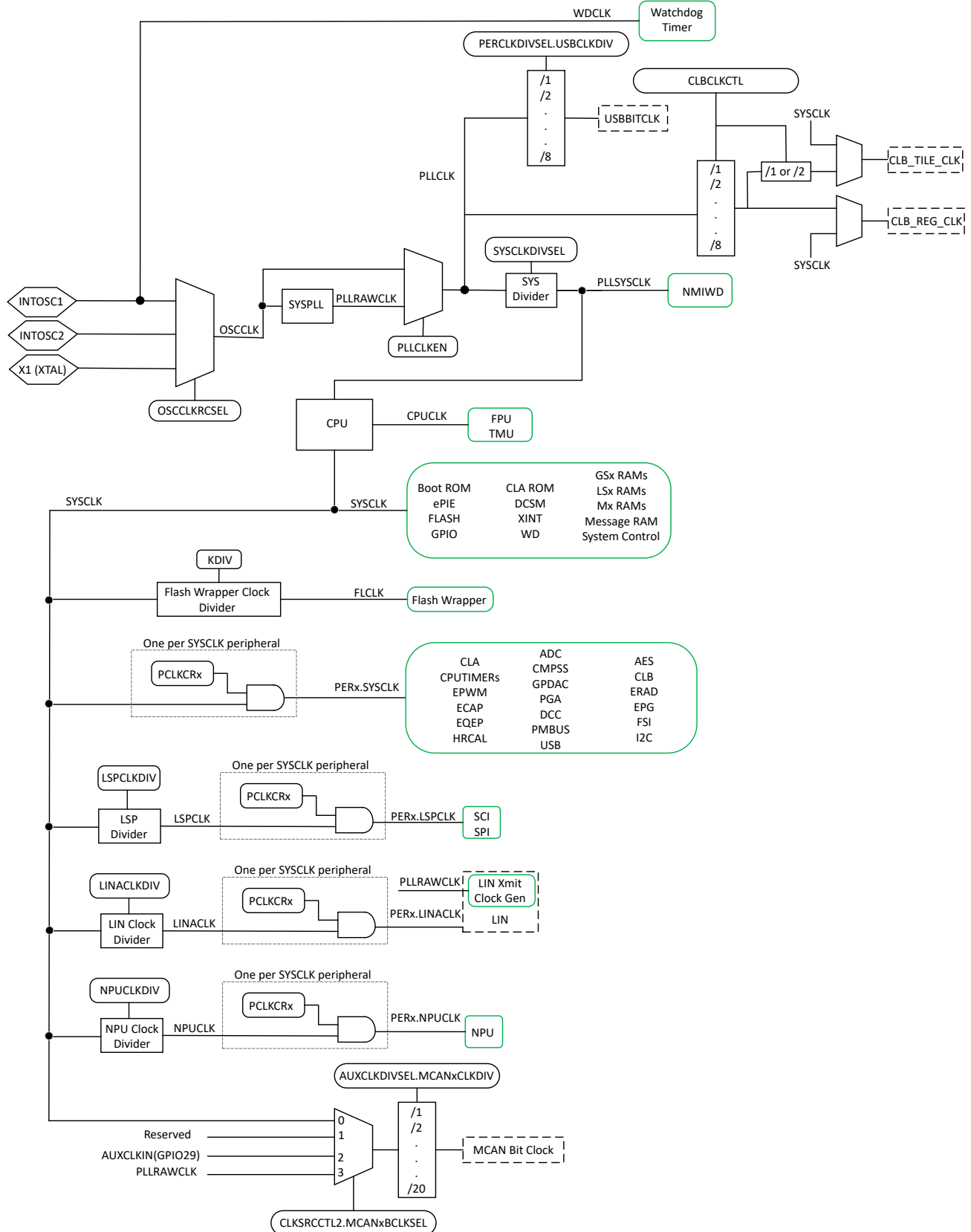
图 6-9. 计时系统
