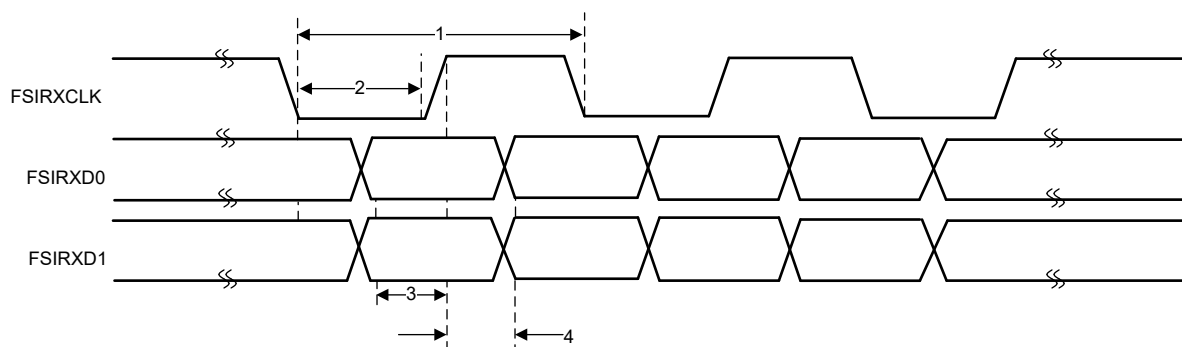
图 6-80. FSIRX 时序
