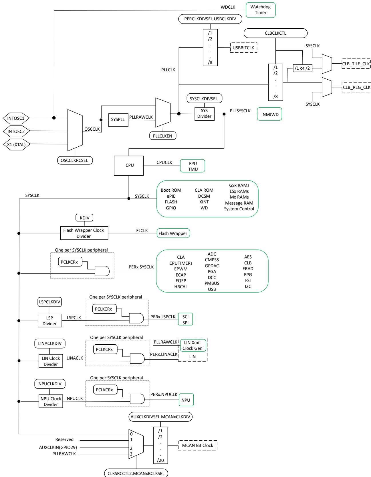
图 6-9. 计时系统
