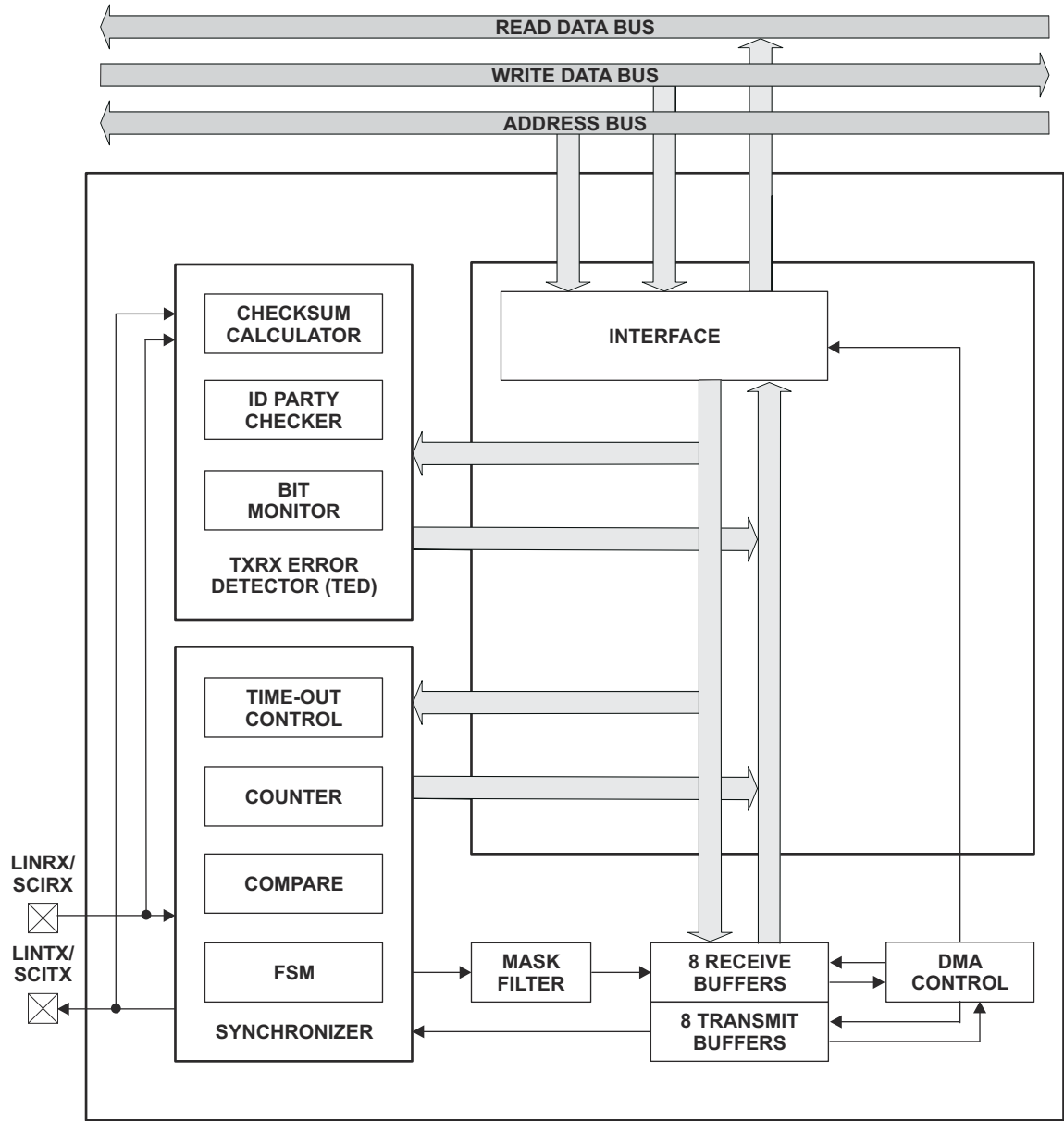
图 6-74. LIN 方框图
