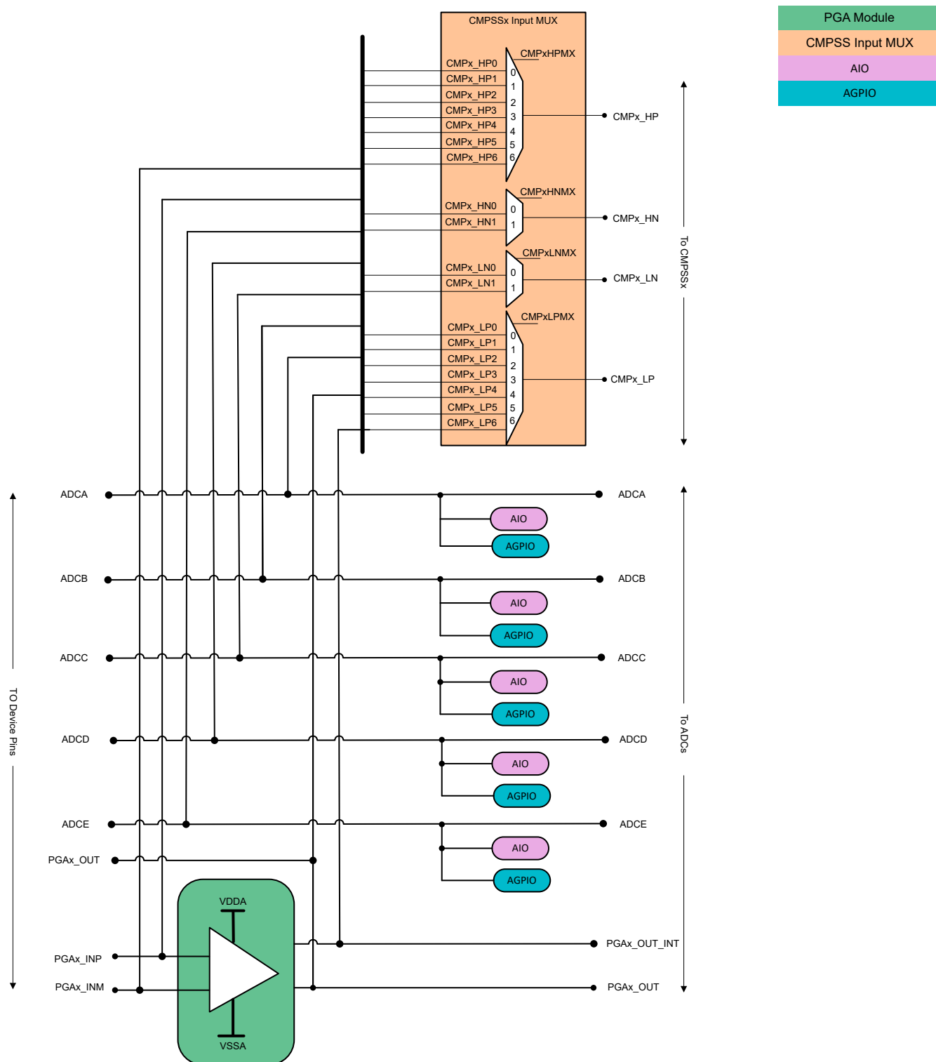
图 6-34. 模拟组连接
