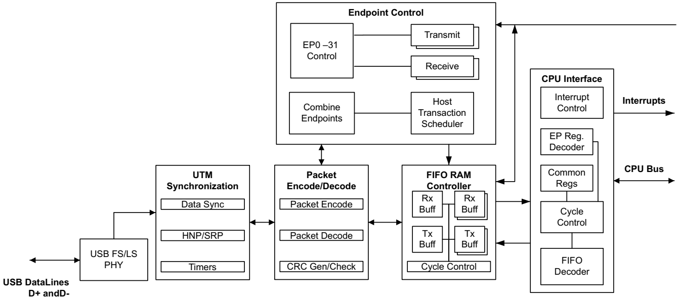
图 6-82. USB 方框图
