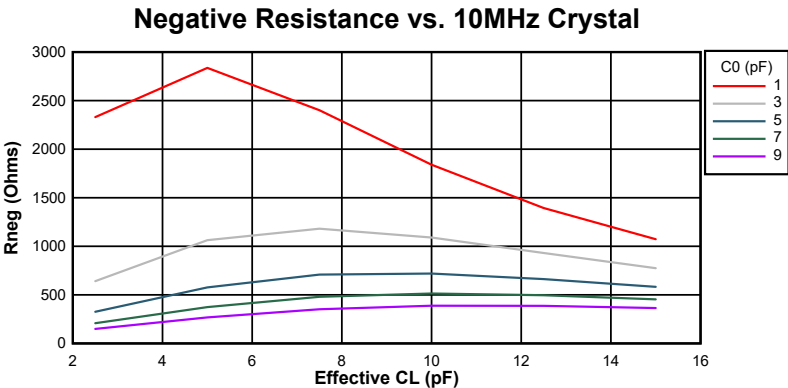
图 6-16. 10MHz 时的负电阻变化
