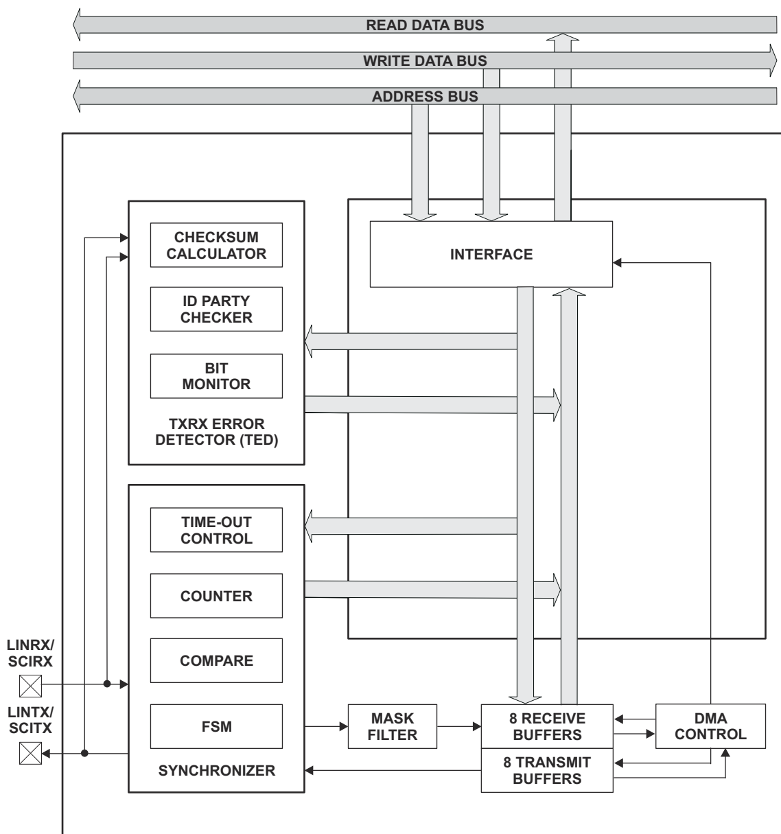
图 6-74. LIN 方框图
