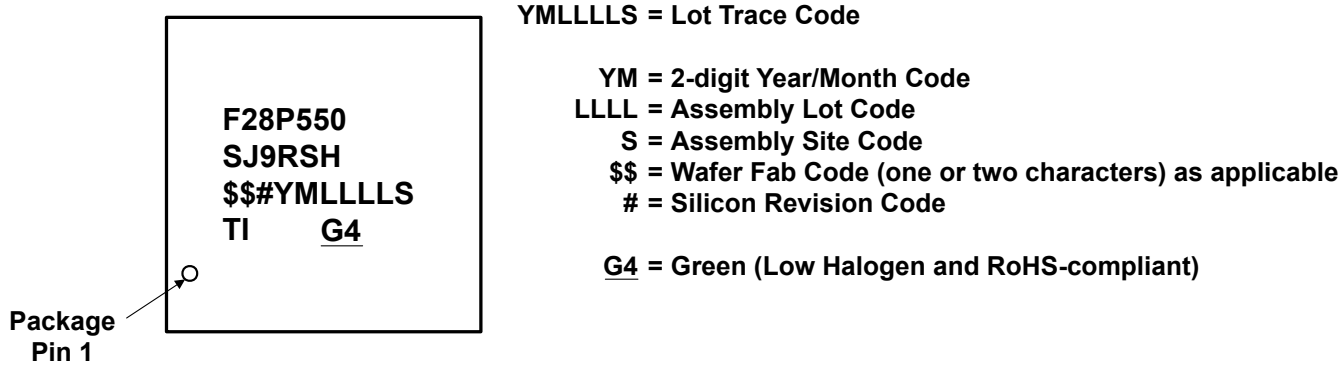
图 9-9. RSH 封装的封装编号法 - 非汽车
