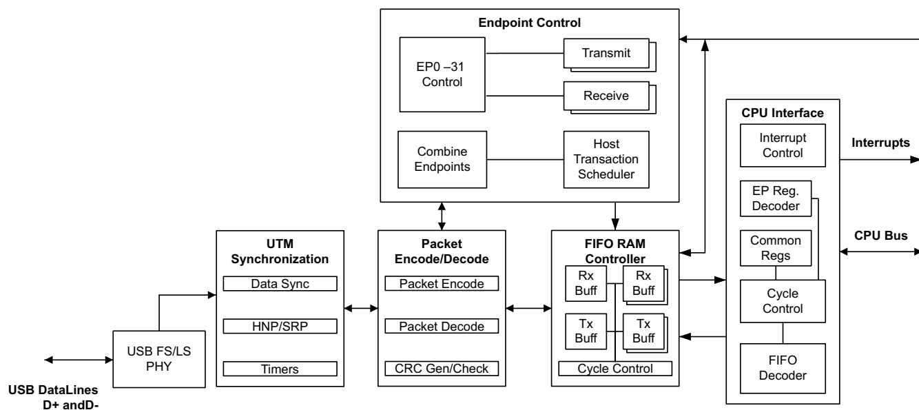
图 7-95. USB 方框图
