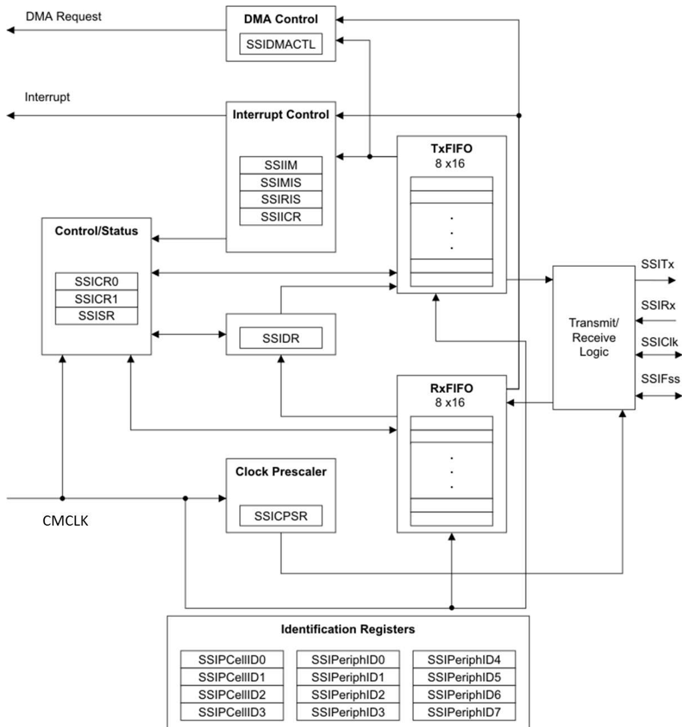
图 7-106. SSI 方框图
