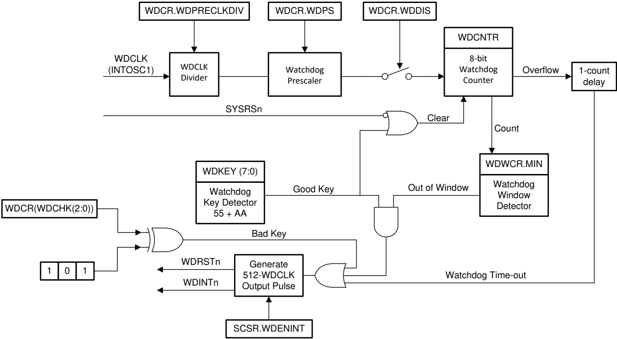
图 8-8. 窗口看门狗
