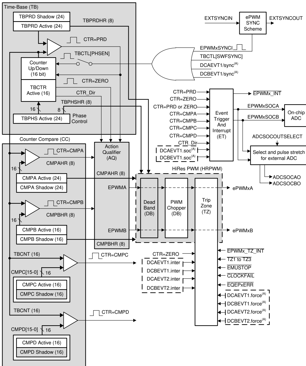
图 7-57. ePWM 子模块和关键内部信号互连
