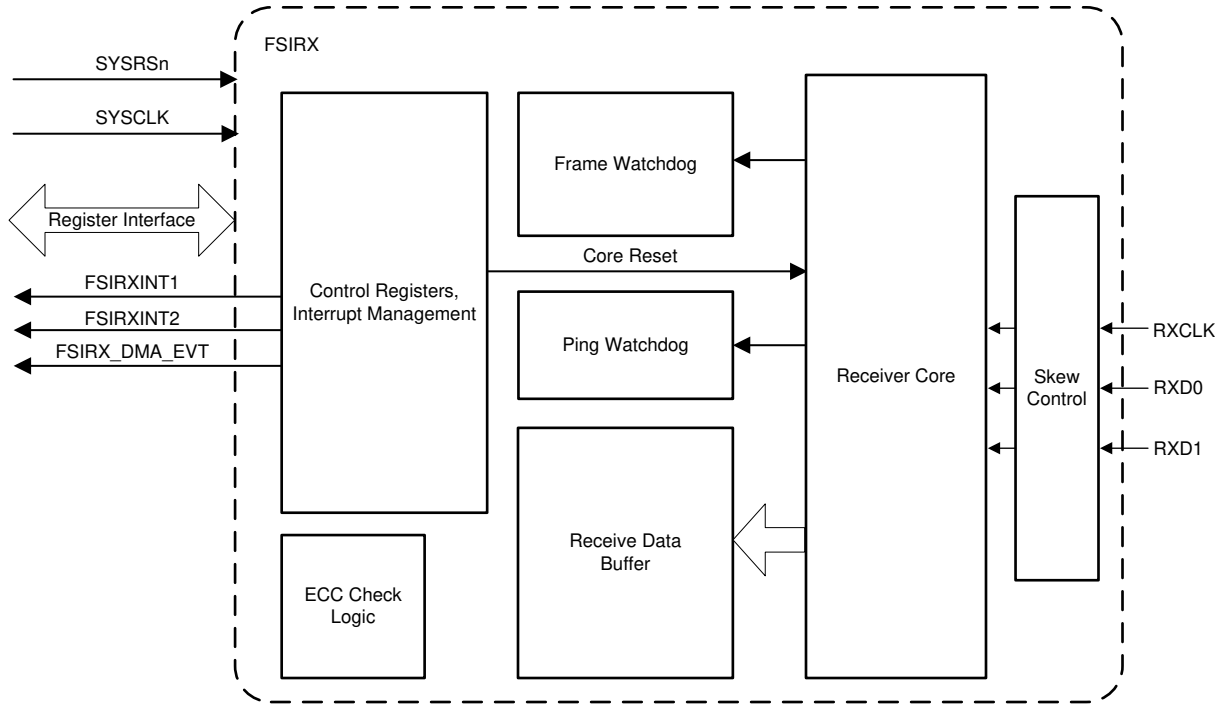
图 7-70. FSIRX 方框图
