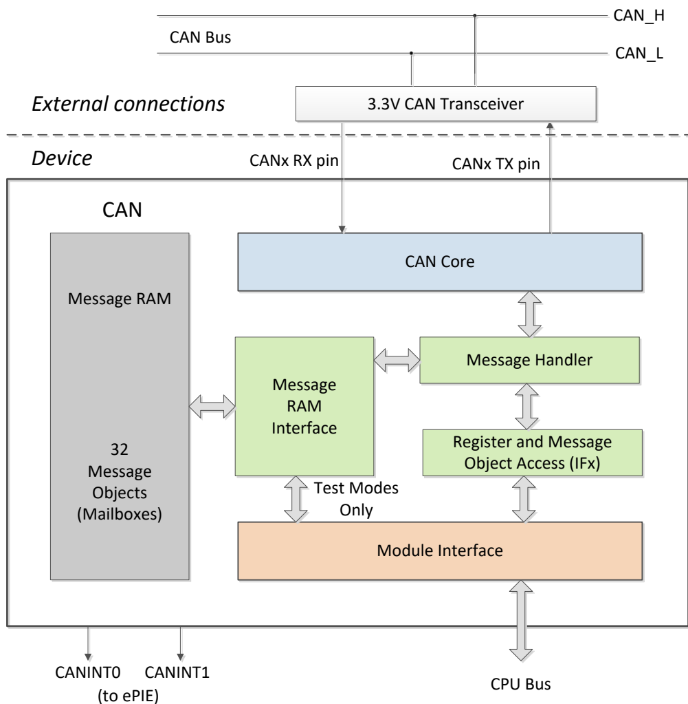
图 7-65. CAN 方框图
