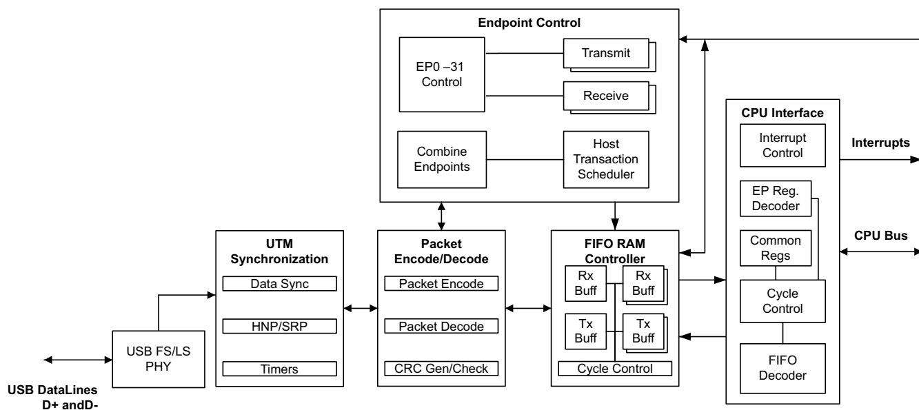
图 7-95. USB 方框图
