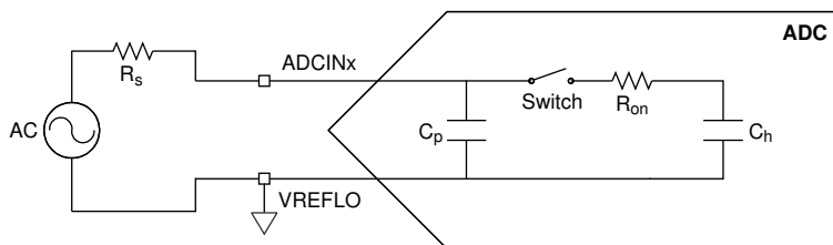
图 7-37. 单端输入模型
