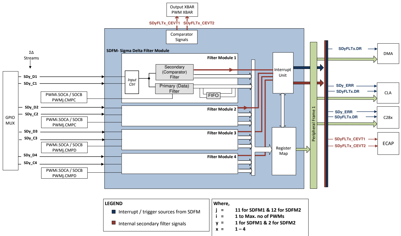
图 7-63. SDFM 方框图
