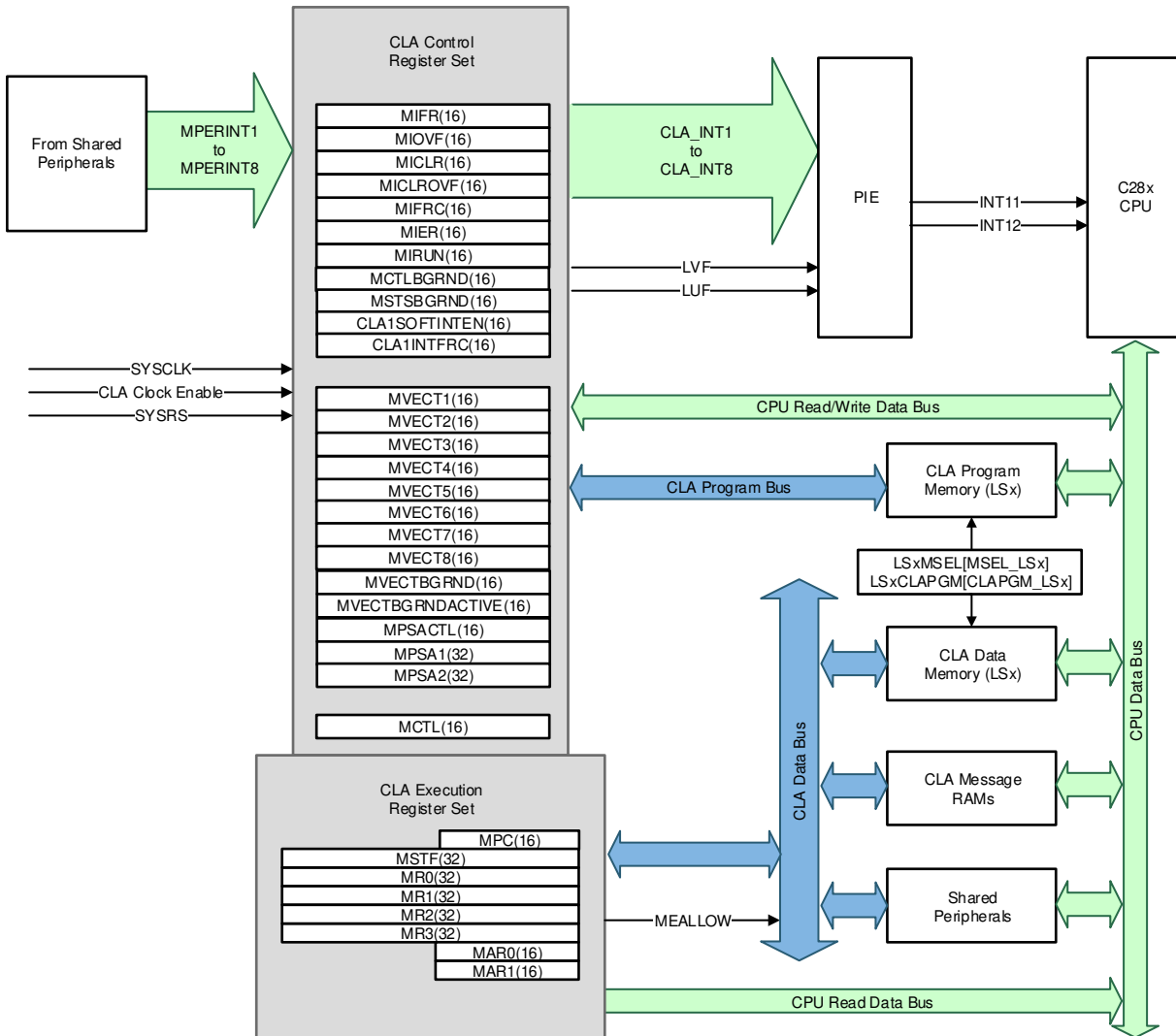
图 8-4. CLA 方框图
