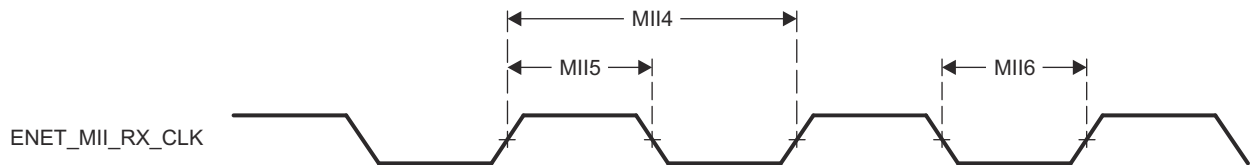
图 7-99. 接收时钟时序 ( MII 运行模式 )
