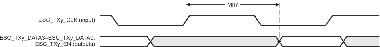
图 7-91. EtherCAT 发送接口时序 ( MII 运行模式 )
