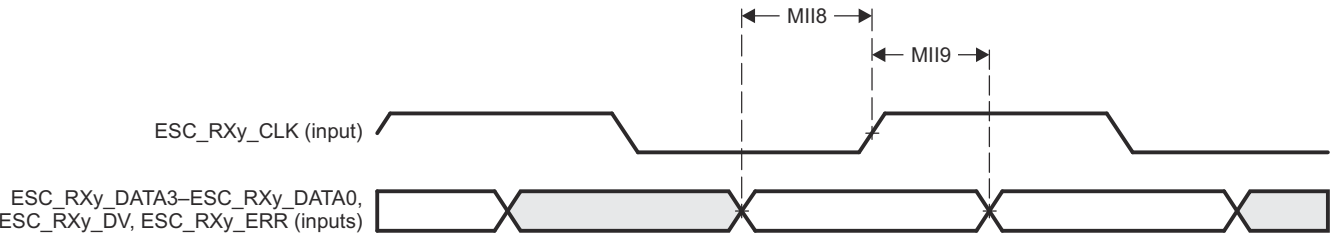
图 7-93. EtherCAT 接收接口时序 ( MII 运行模式 )
