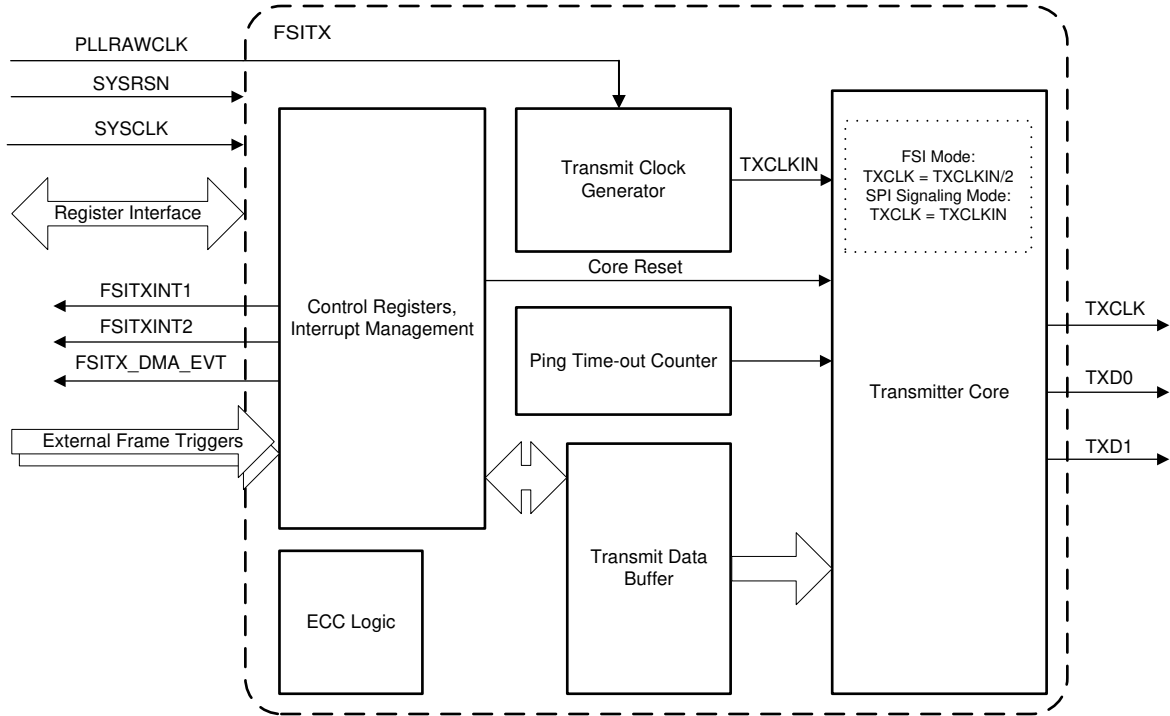
图 7-67. FSITX 方框图
