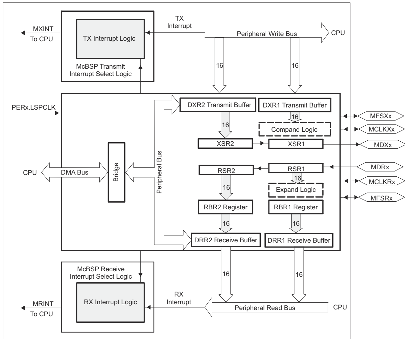
图 6-68. McBSP 方框图
