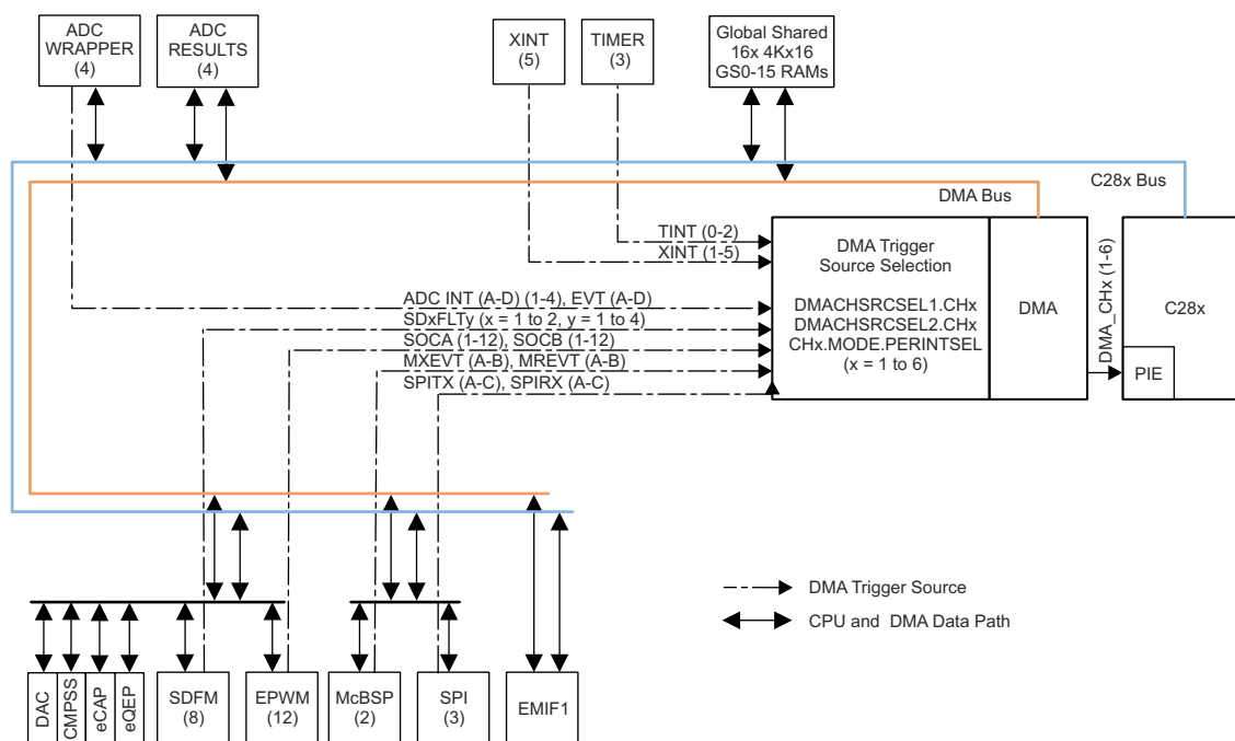
图 7-3. DMA 方框图
