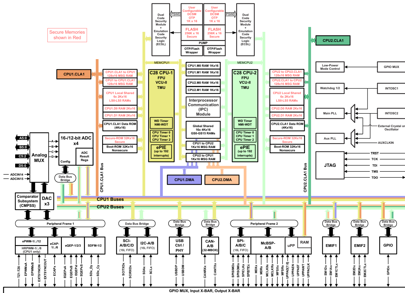
图 3-1. 功能方框图
