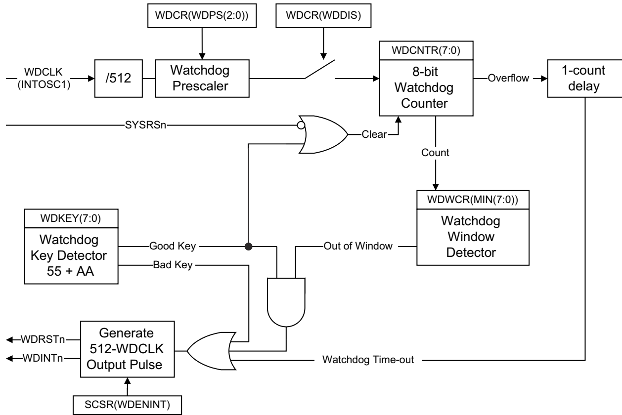
图 7-5. 窗口看门狗
