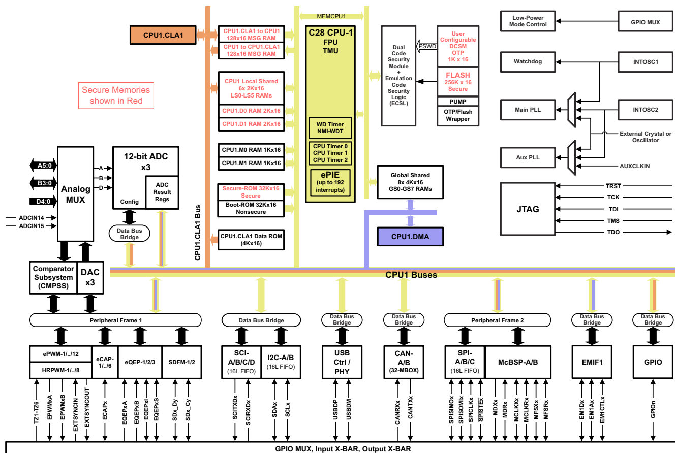
图 3-1. 功能方框图
