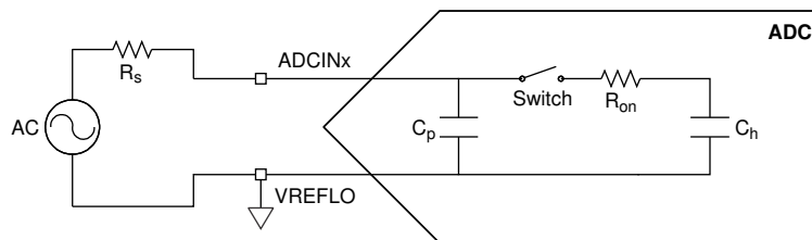
图 6-35. 单端输入模型
