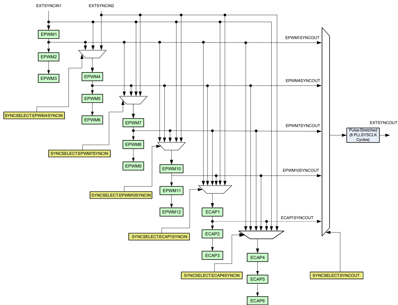
图 6-52. 同步链架构
