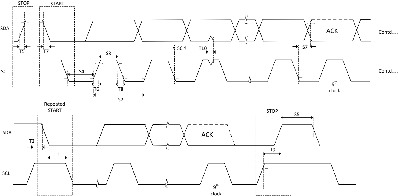
图 6-63. I2C 时序图
