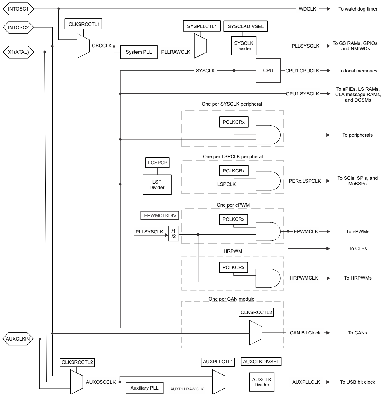
图 6-7. 计时系统
