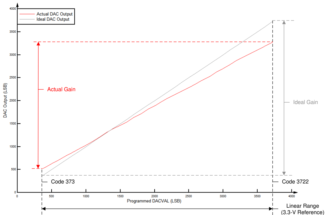
图 6-46. 缓冲 DAC 增益
