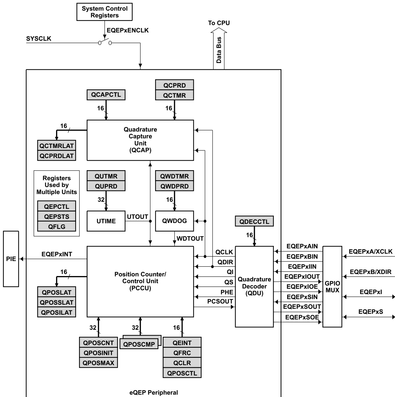
图 6-55. eQEP 方框图
