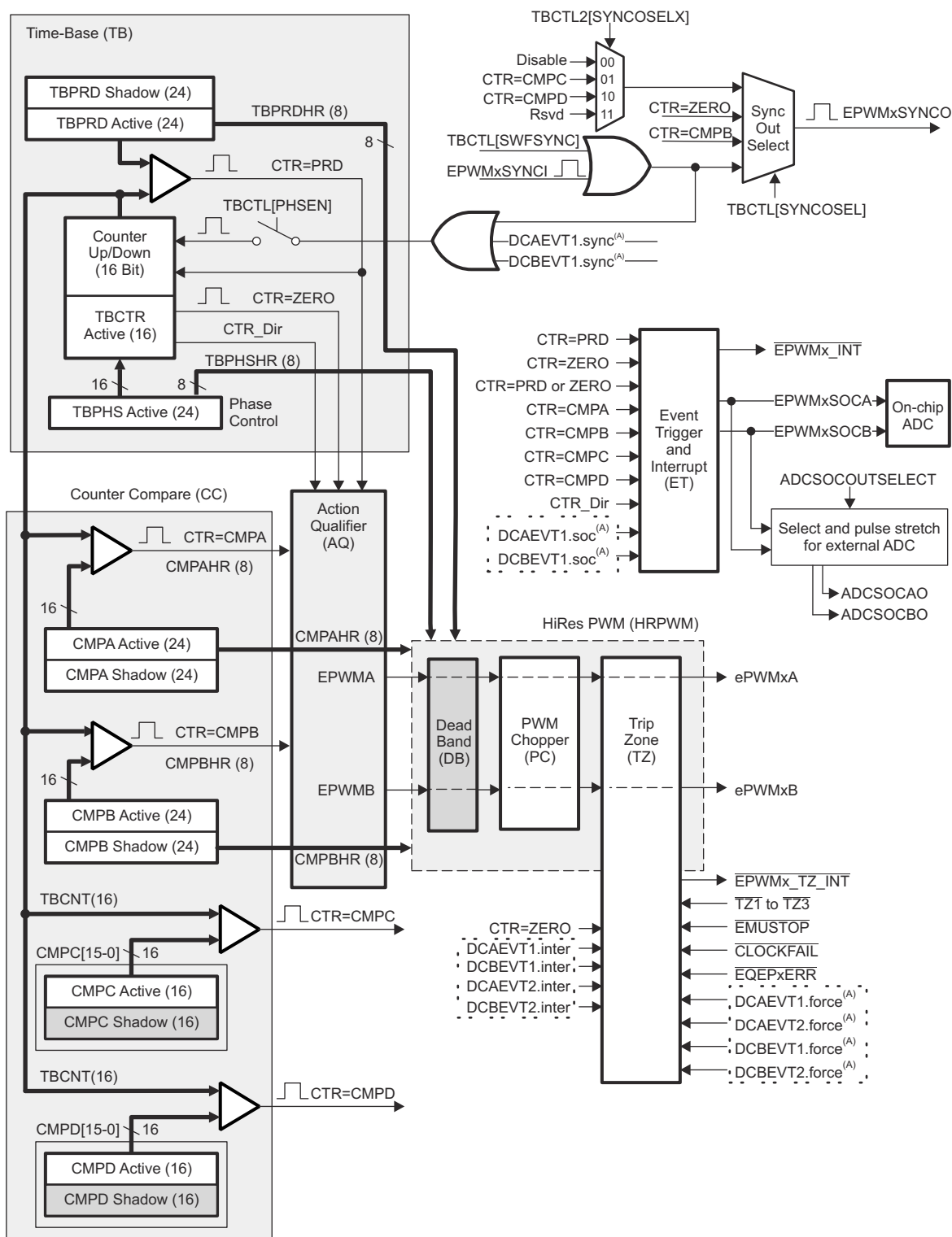
图 6-50. ePWM 子模块和关键内部信号互连
