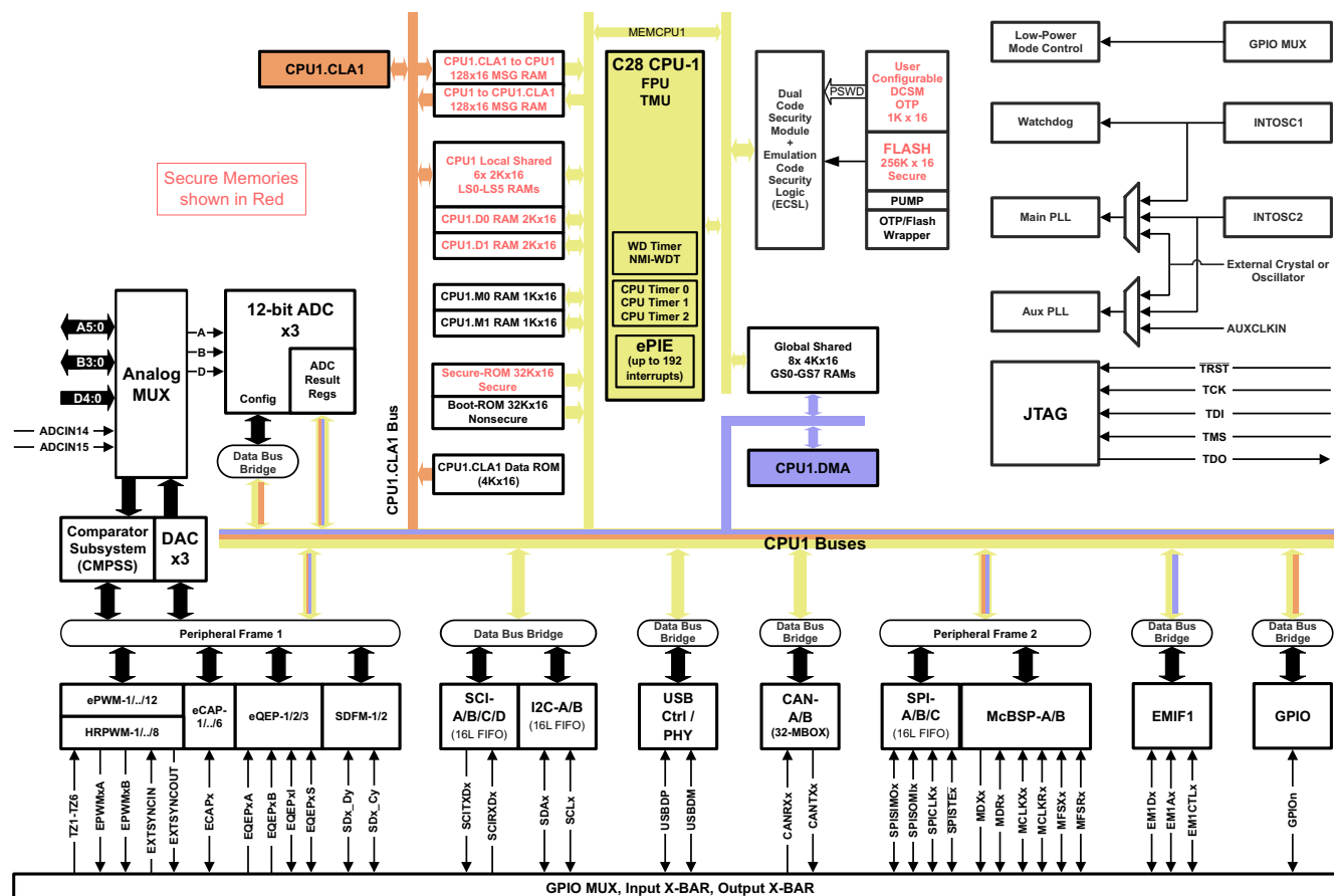
图 7-1. 功能方框图
