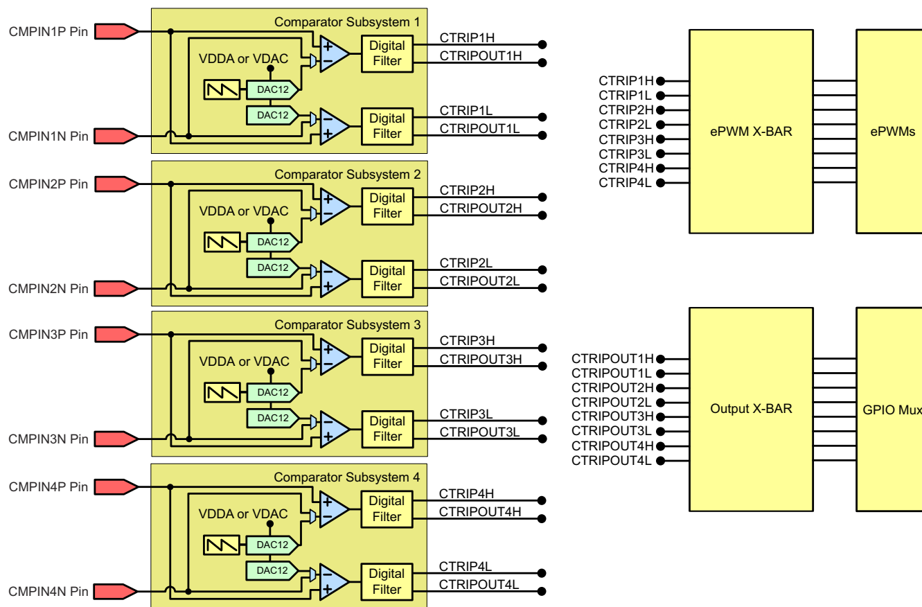
图 6-38. CMPSS 连接 ( 100 引脚 PZP )
