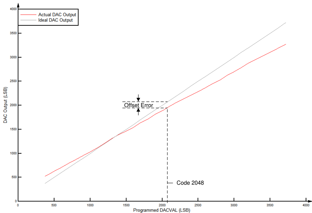
图 6-45. 缓冲 DAC 偏移
