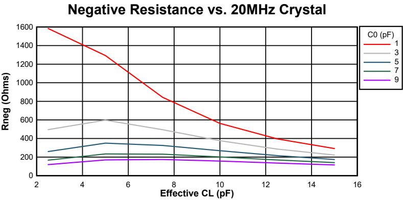
图 6-12. 20 MHz 时的负电阻变化
