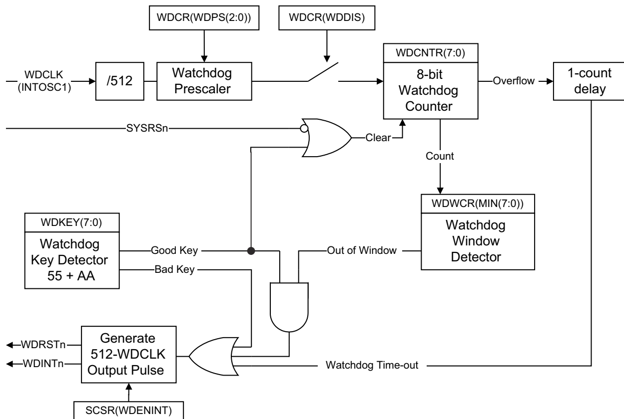
图 7-4. 窗口看门狗
