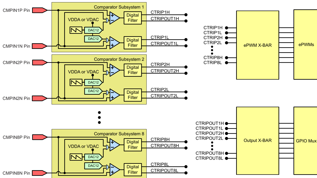
图 6-37. CMPSS 连接 ( 176 引脚 PTP )
