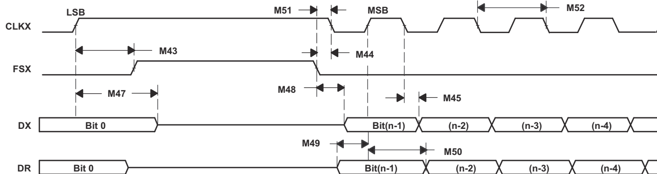
图 6-69. McBSP 时序作为 SPI 主器件或从器件：CLKSTP=10b，CLKXP=1
