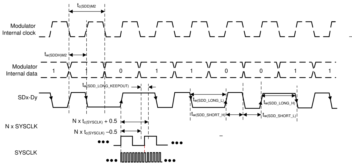
图 6-59. SDFM 时序图 - 模式 2
