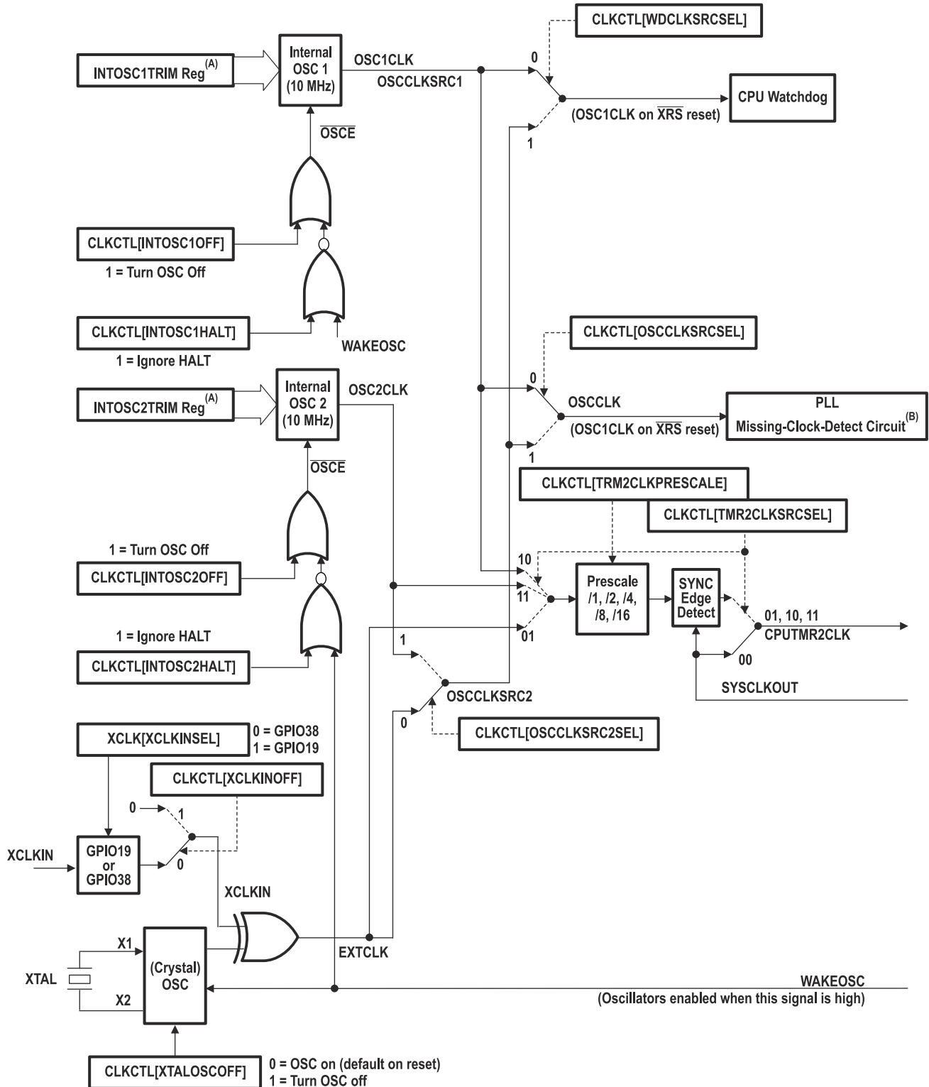
图 8-7. Clock Tree
