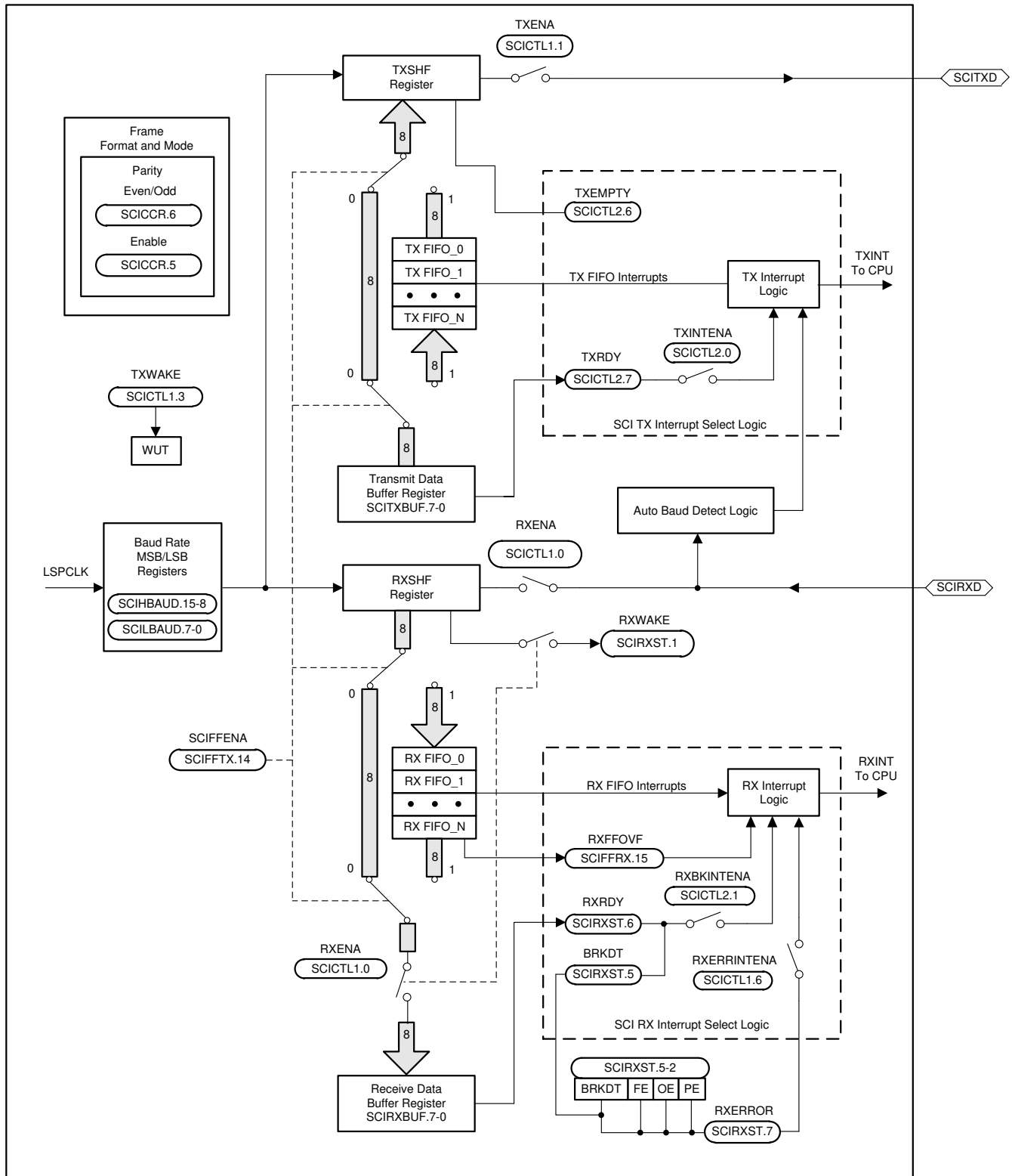
图 8-33. SCI Module Block Diagram
