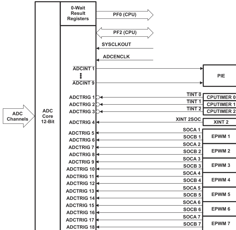
图 8-16. ADC Connections
