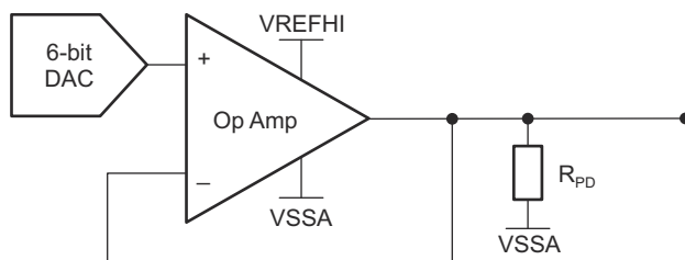
图 8-26. V_{REFOUT}
