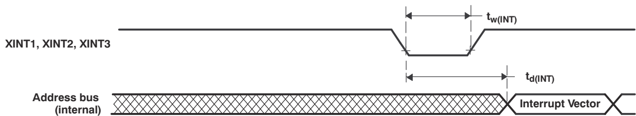
图 7-14. 外部中断时序
