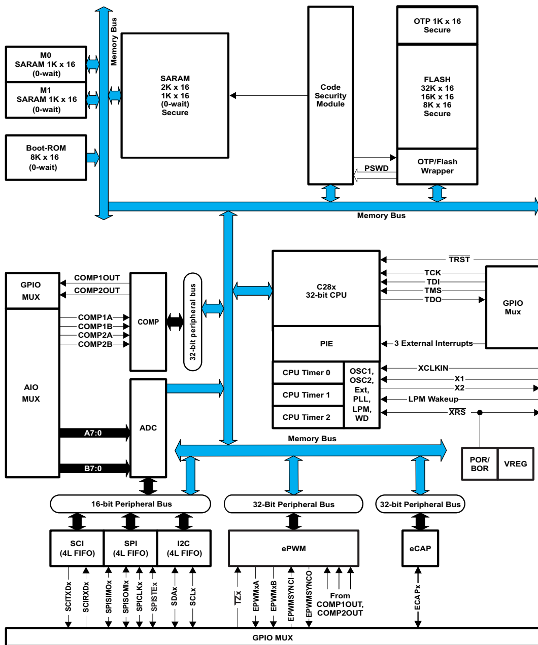
图 1-1. 功能框图
