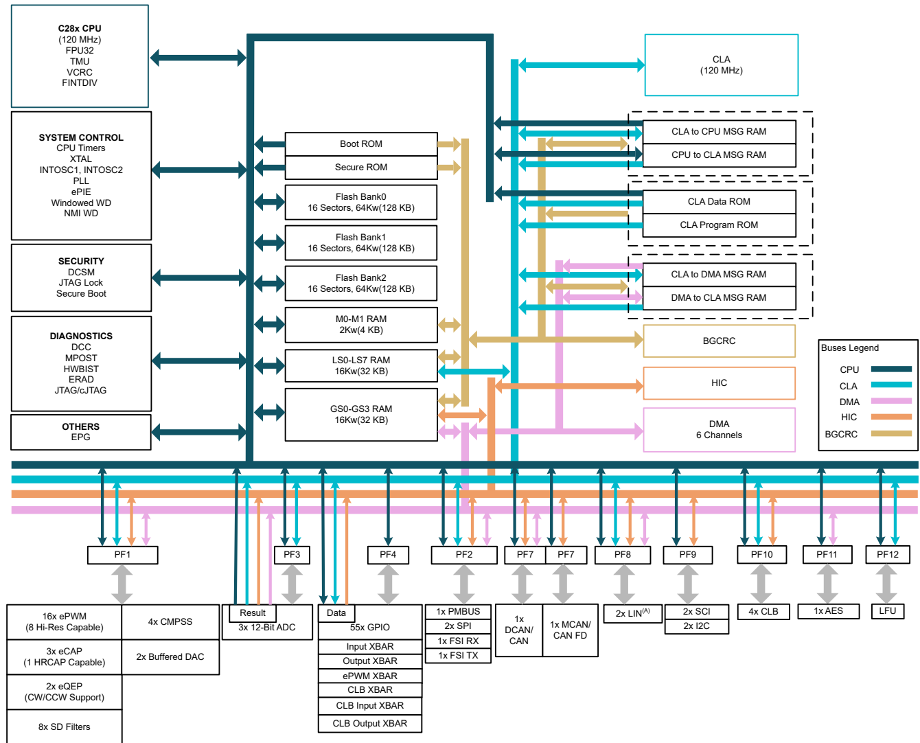
图 3-1. 功能方框图
