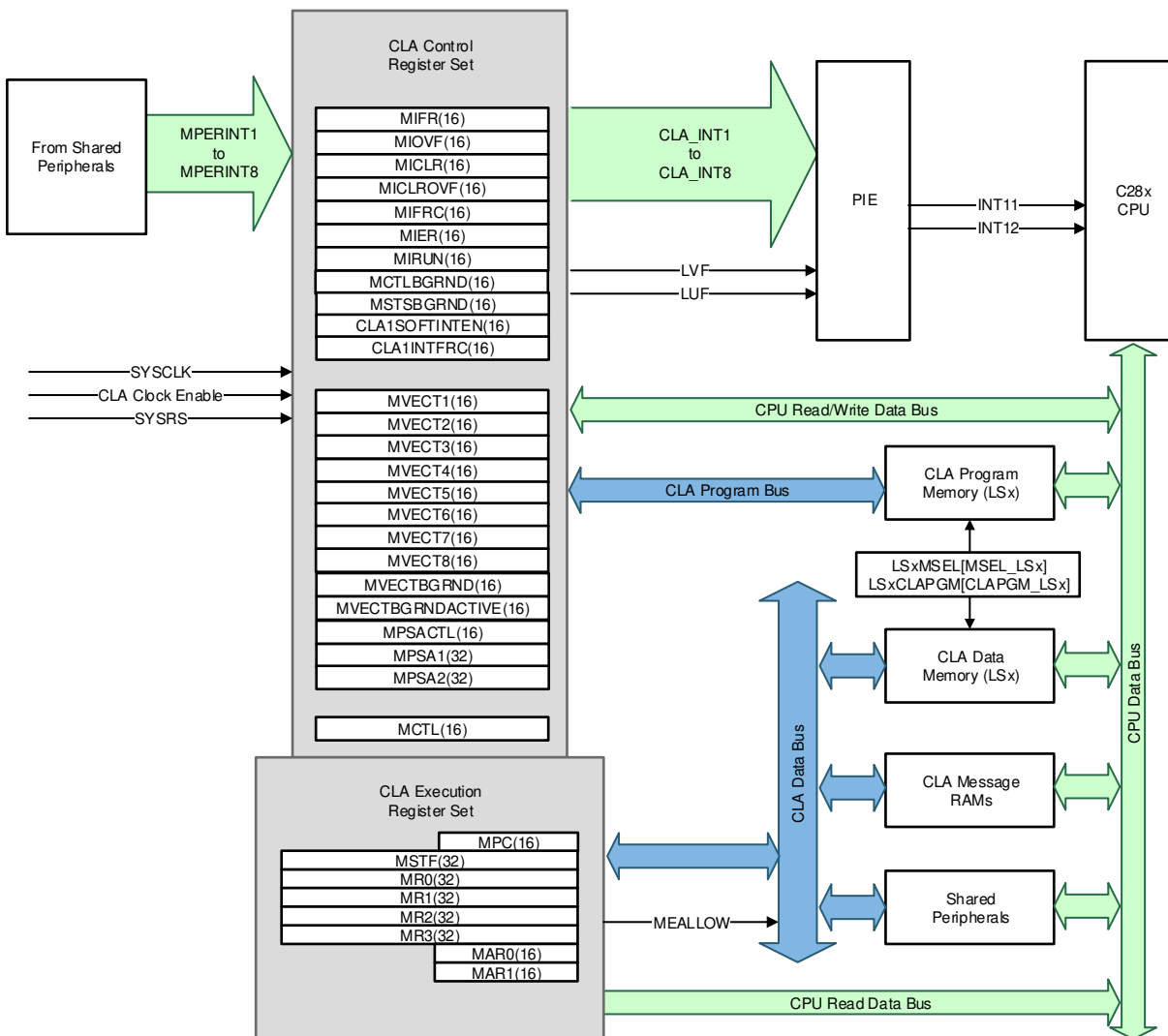
图 7-2. CLA 方框图
