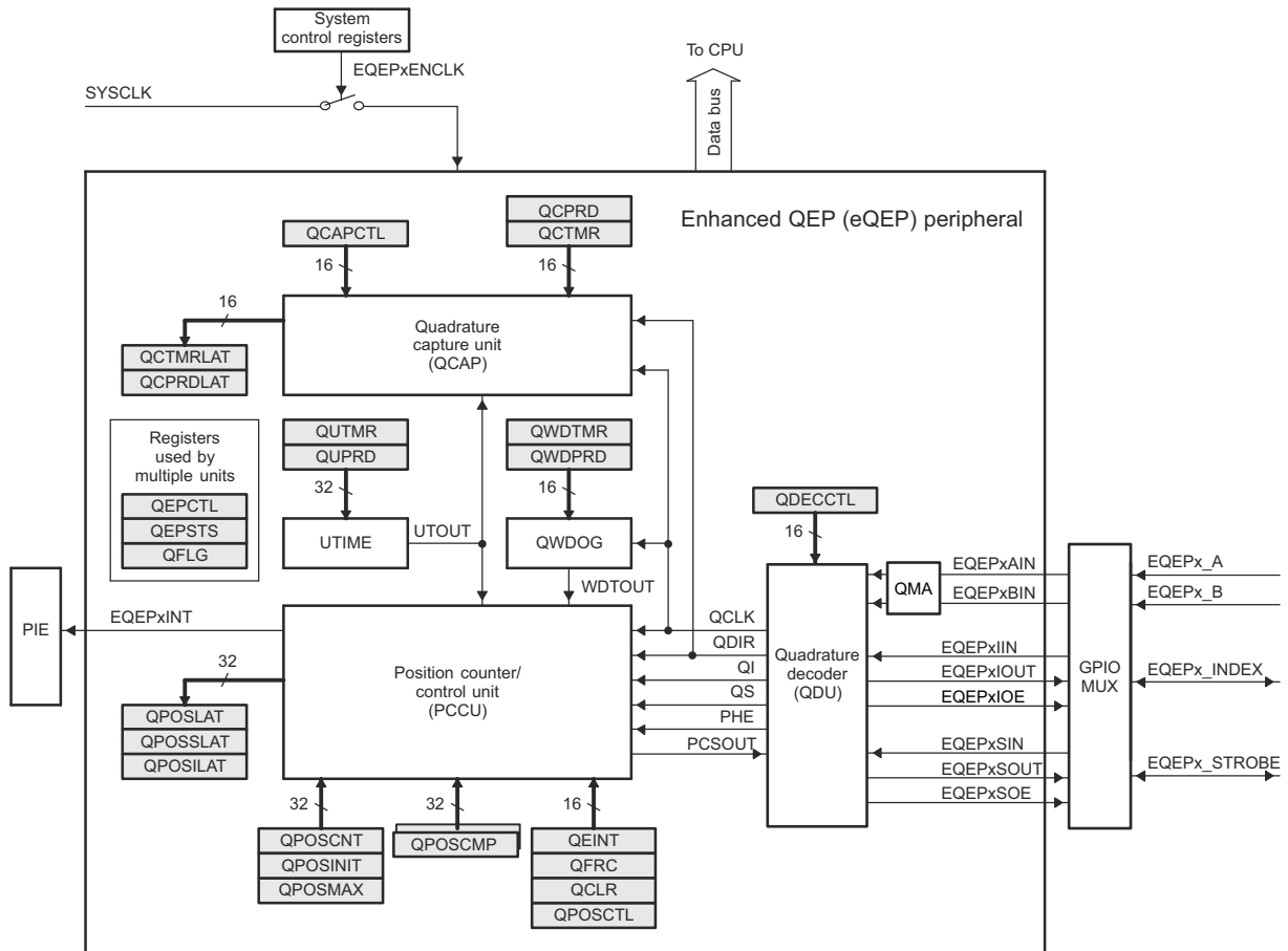
图 6-64. eQEP 方框图
