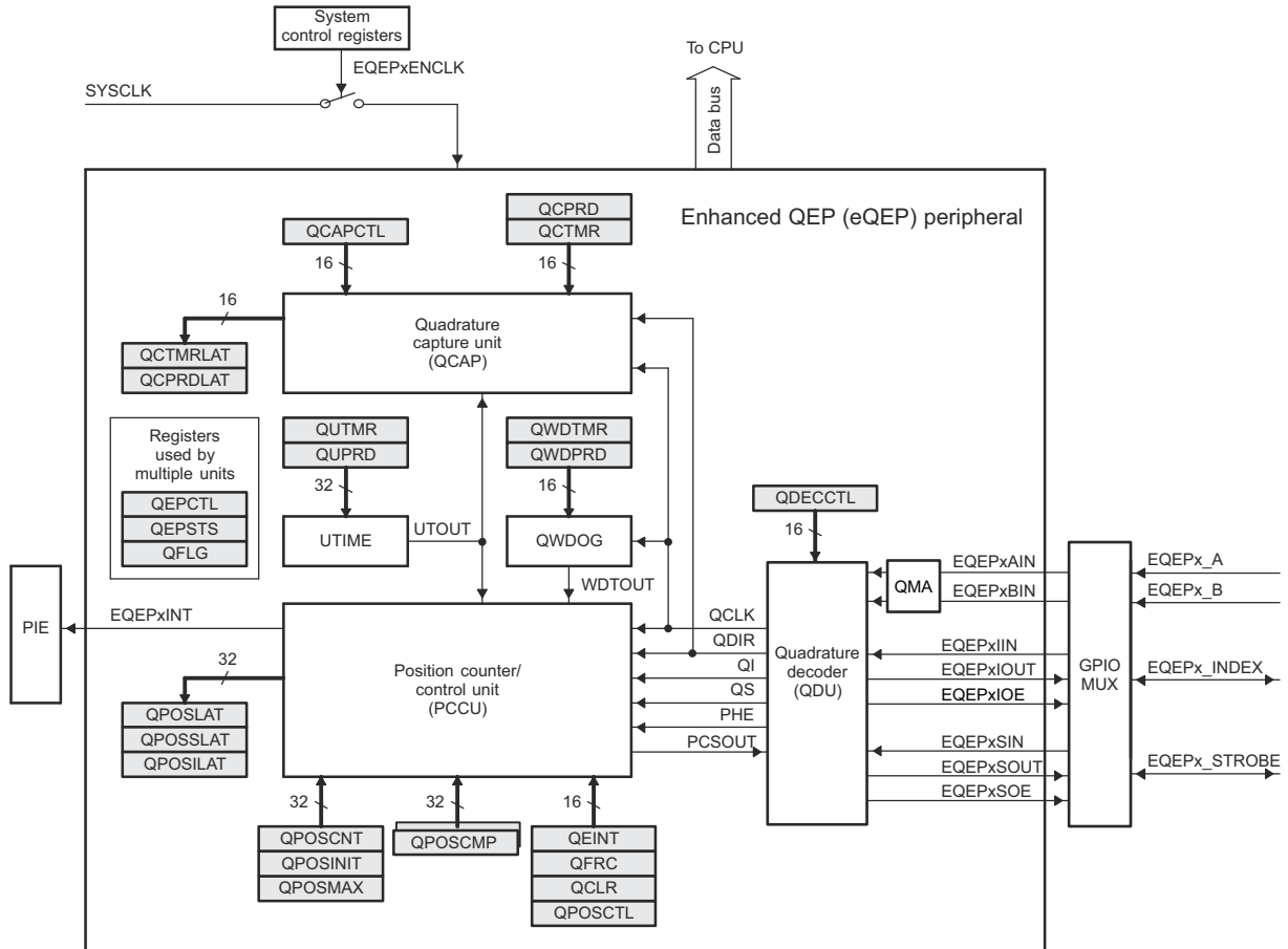
图 6-64. eQEP 方框图
