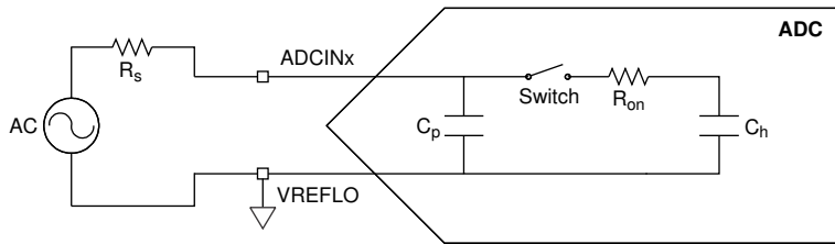
图 6-44. 输入模型
