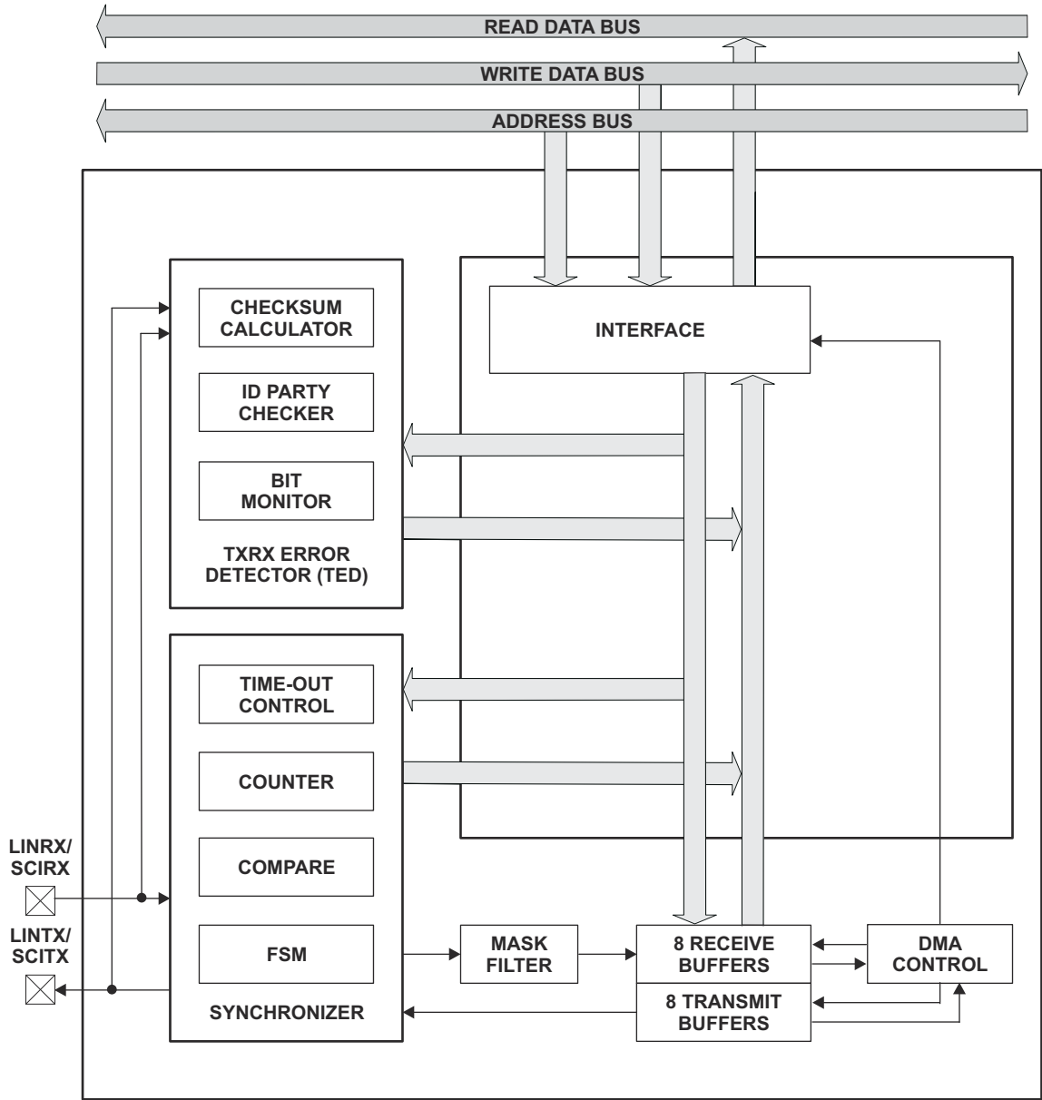
图 6-77. LIN 方框图
