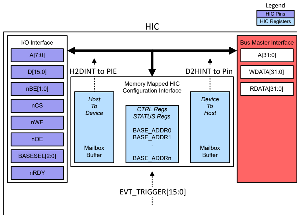
图 6-85. HIC 方框图
