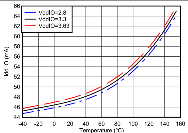
图 6-3. 工作电流与温度间的关系
