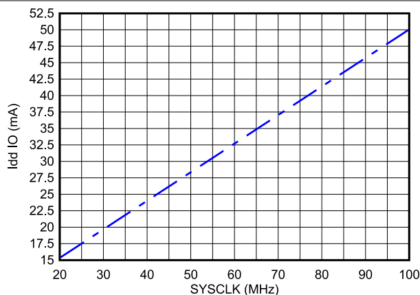
图 6-2. 工作电流与频率间的关系
