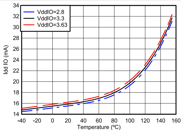
图 6-4. 电流与温度间的关系 - IDLE 模式
