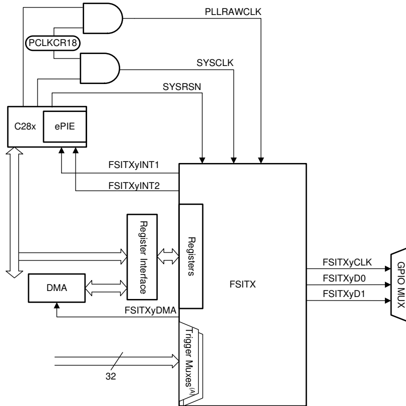
图 6-71. FSITX CPU 接口
