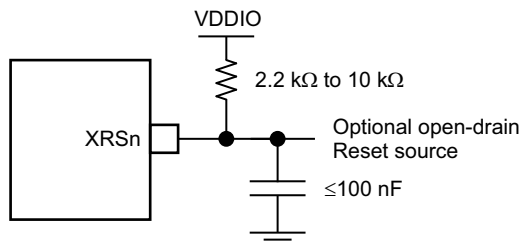
图 6-10. 复位电路
