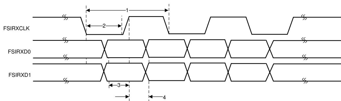
图 6-76. FSIRX 时序
