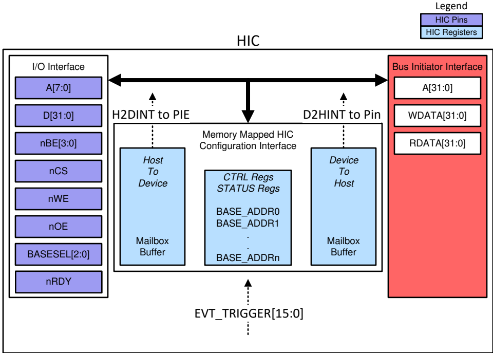
图 6-78. HIC 方框图
