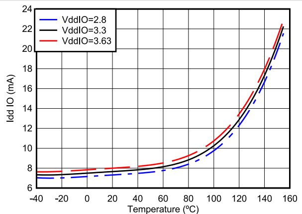
图 6-5. 电流与温度间的关系 - STANDBY 模式
