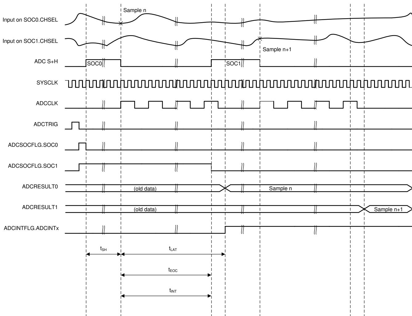
图 6-43. ADC 时序
