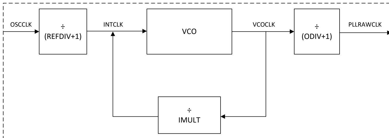
图 6-14. 系统 PLL
