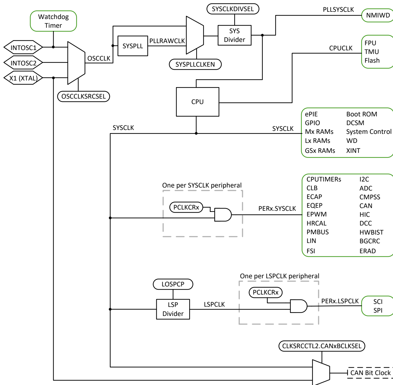
图 6-13. 计时系统
