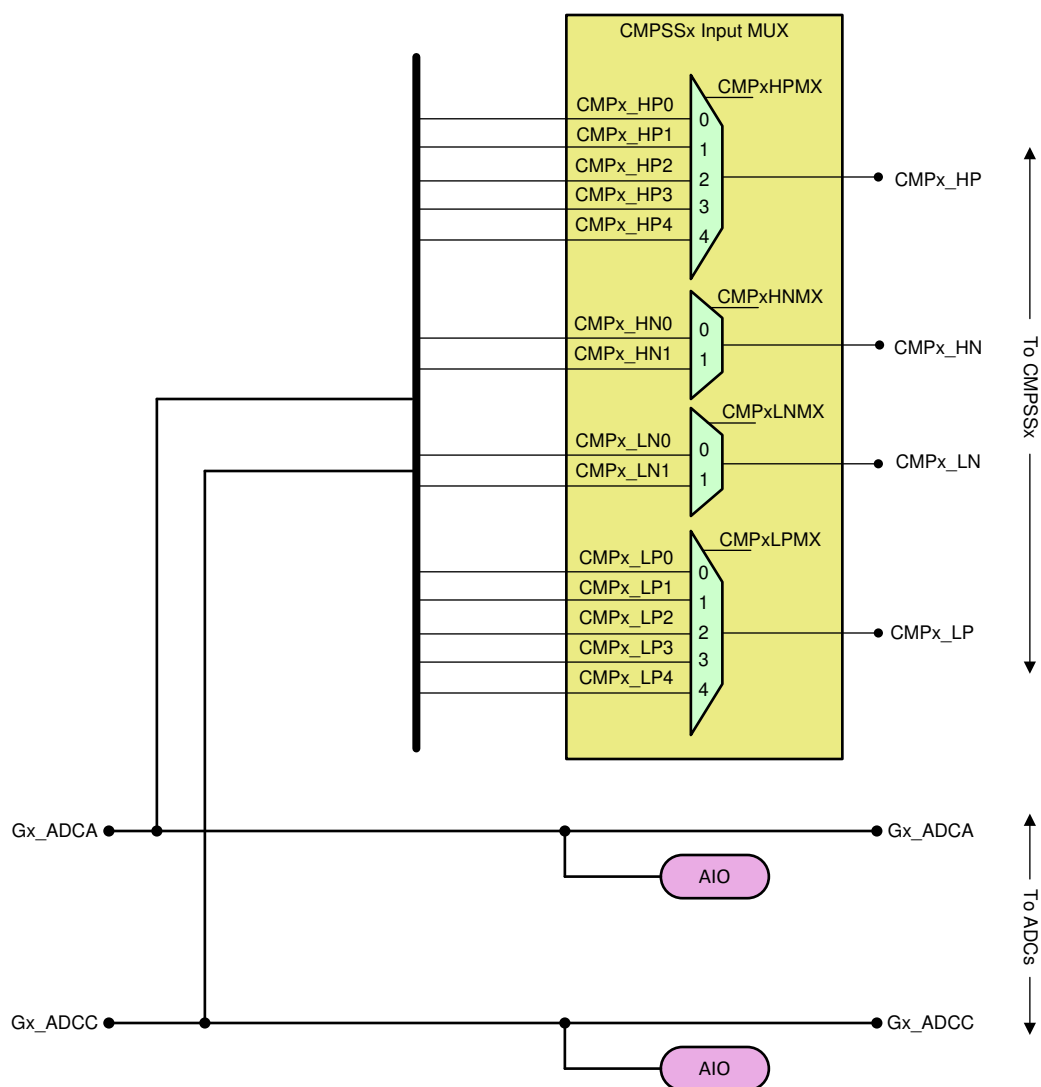
图 6-38. 模拟组连接
