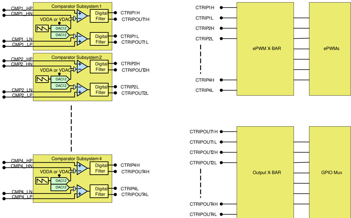
图 6-44. CMPSS 连接
