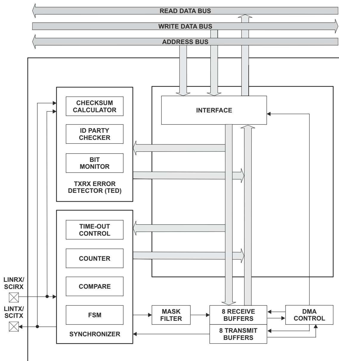
图 6-70. LIN 方框图
