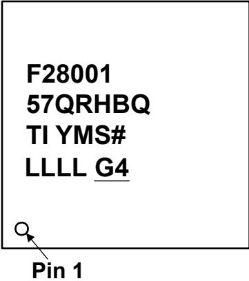
图 9-9. RHB 封装的封装编号法 ( 通过 AEC-Q100 1 级认证 )
