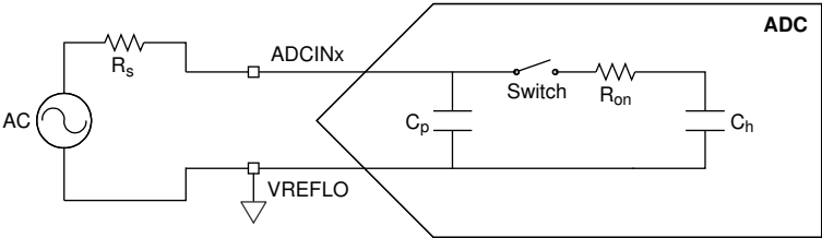
图 6-41. 输入模型
