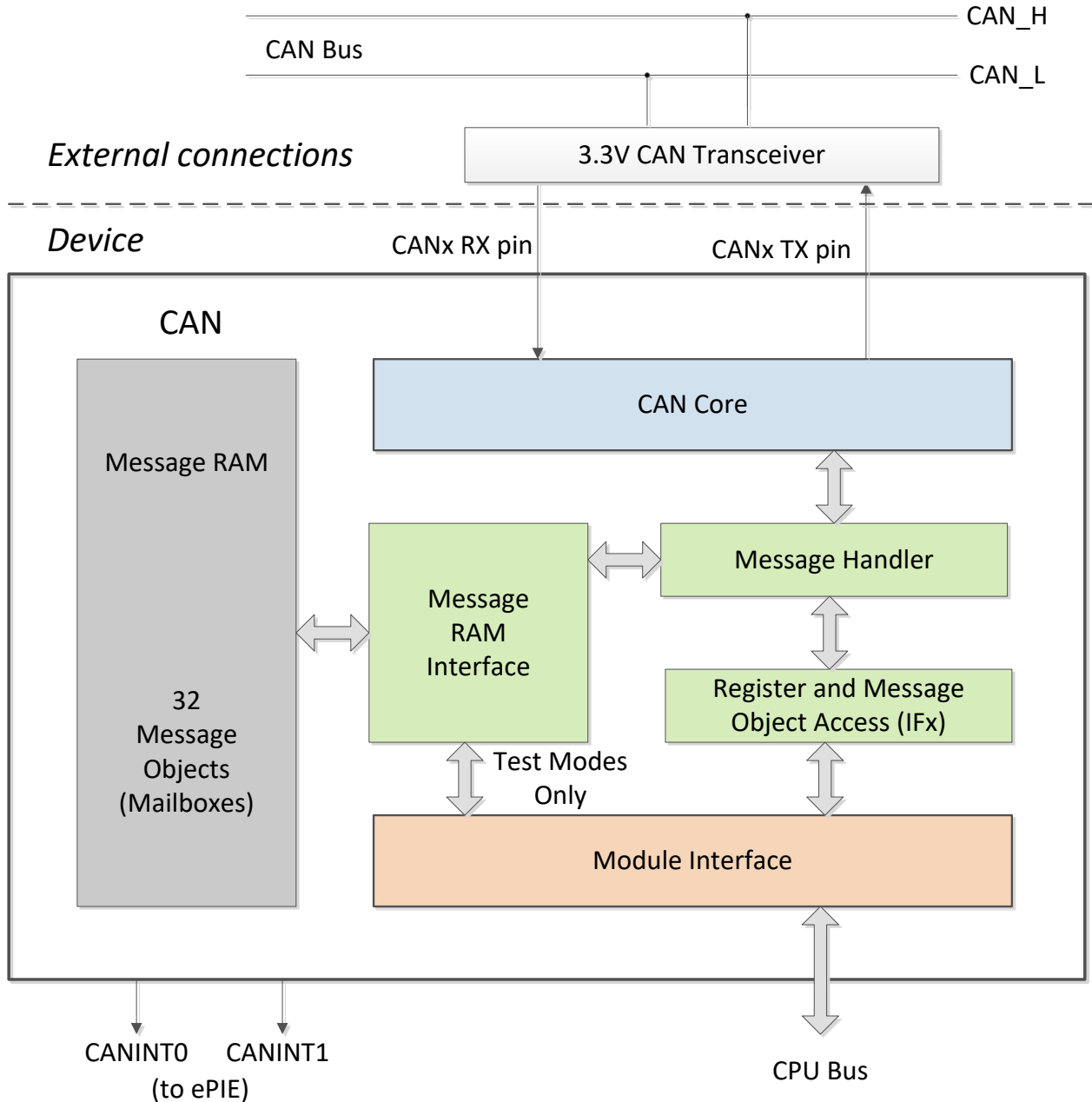
图 6-61. CAN 方框图
