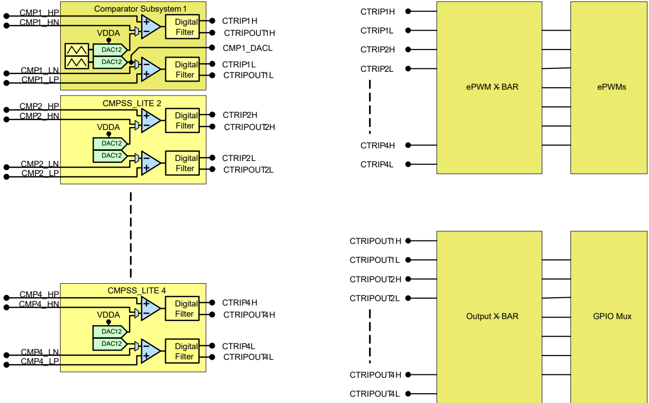
图 6-43. CMPSS 连接
