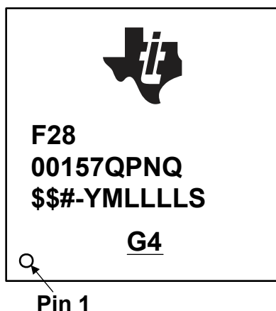
图 9-3. PN 封装的封装编号法 ( 通过 AEC-Q100 1 级认证 )
