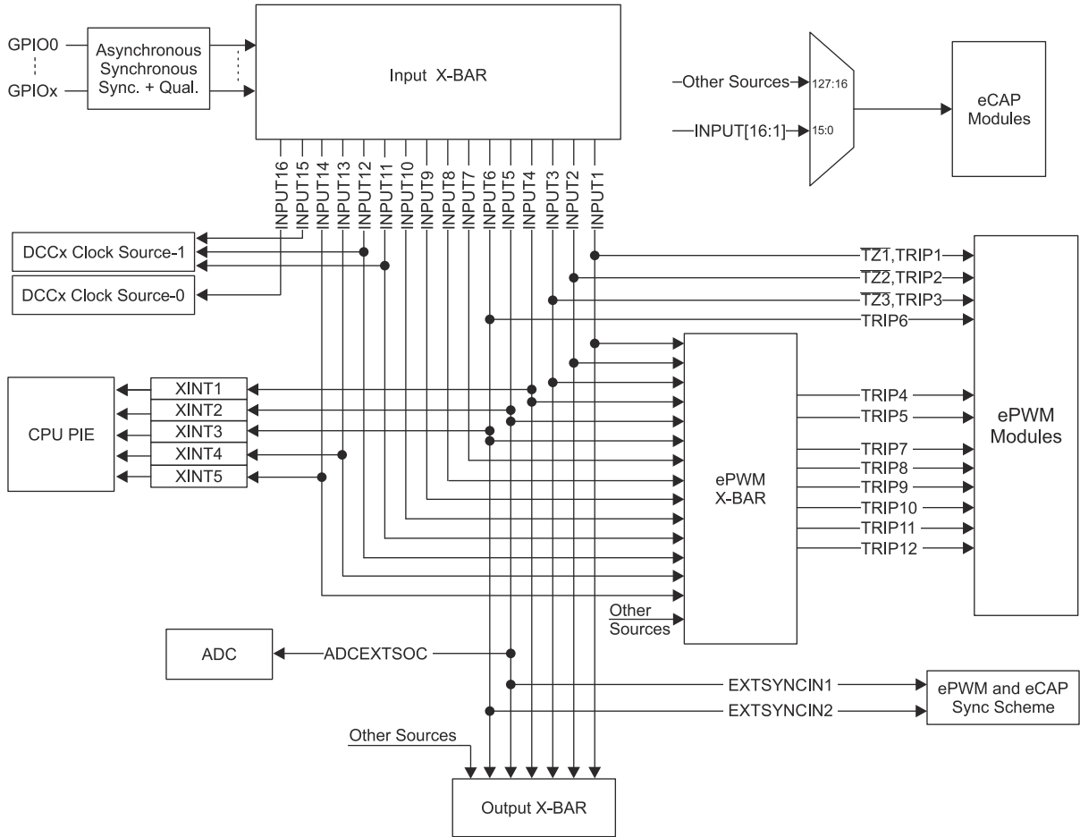
图 5-6. 输入 X-BAR
