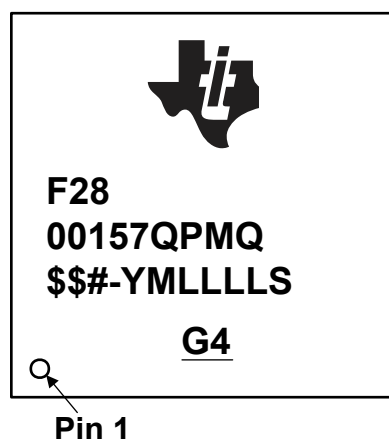
图 9-5. PM 封装的封装编号法 ( 通过 AEC-Q100 1 级认证 )
