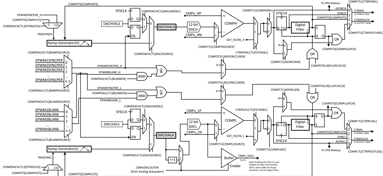
图 6-44. CMPSS 模块方框图
