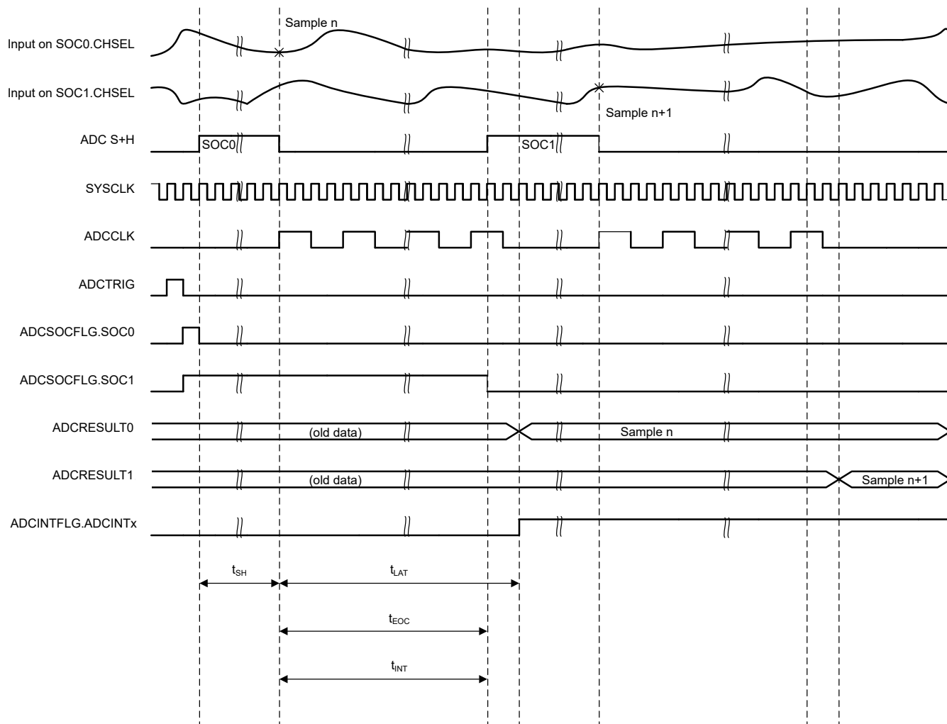
图 6-42. ADC 时序
