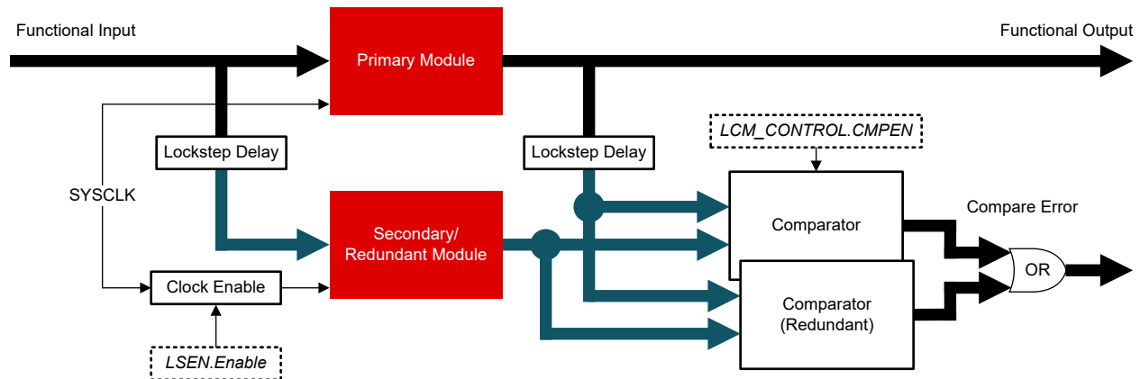
图 7-2. LCM 方框图
