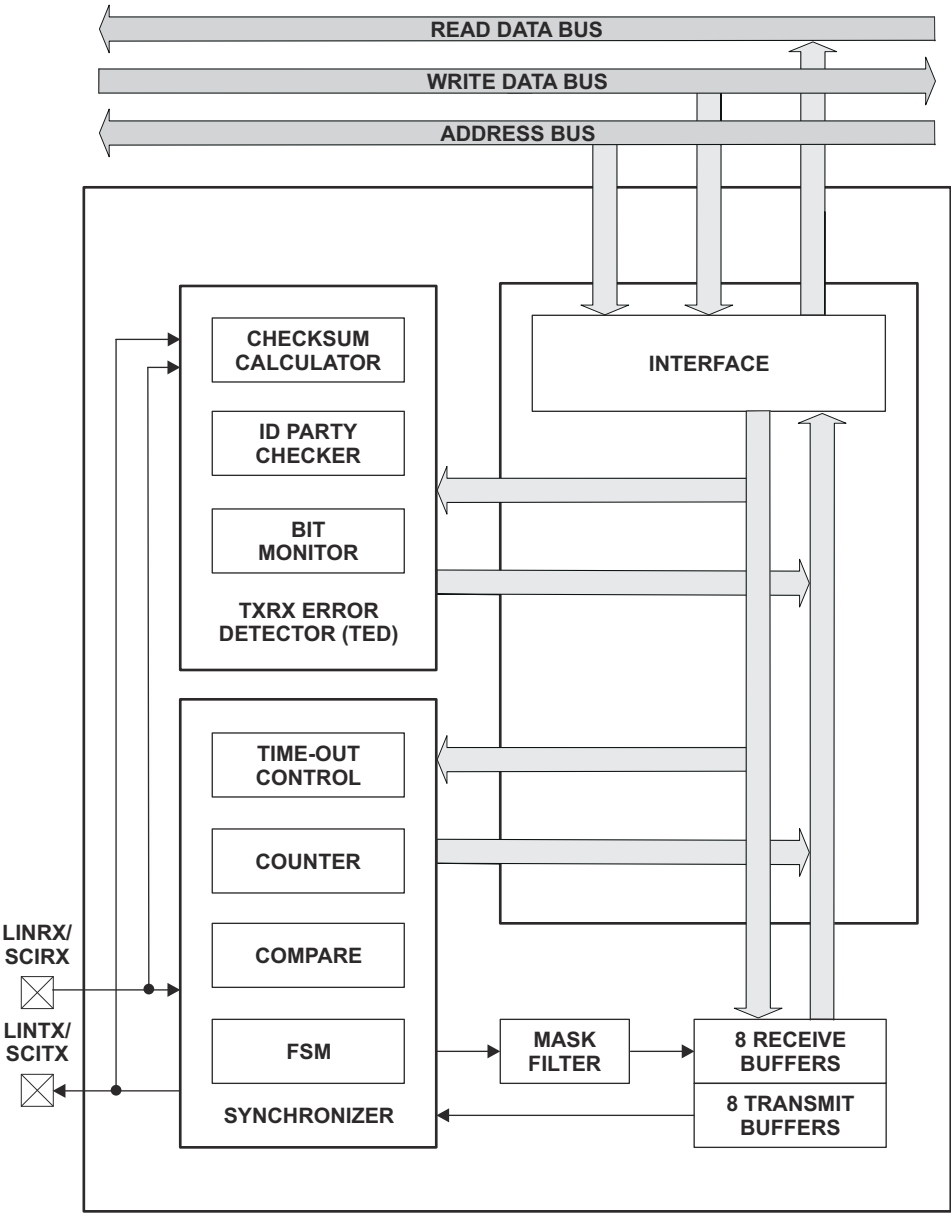
图 6-72. LIN 方框图
