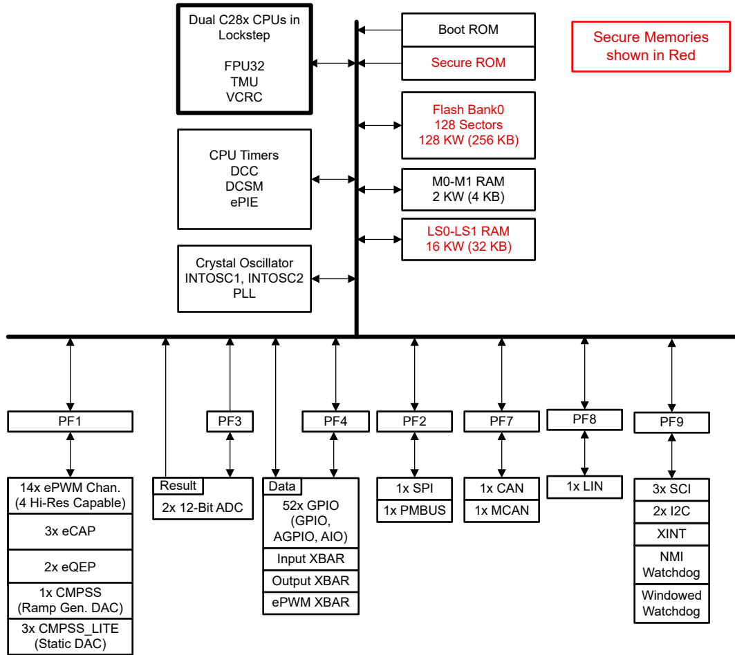
图 7-1. 功能方框图
