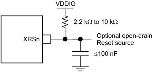
图 6-8. 复位电路
