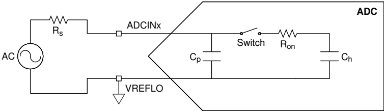
图 6-41. 输入模型
