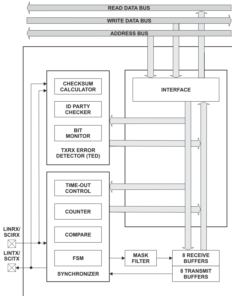
图 6-72. LIN 方框图
