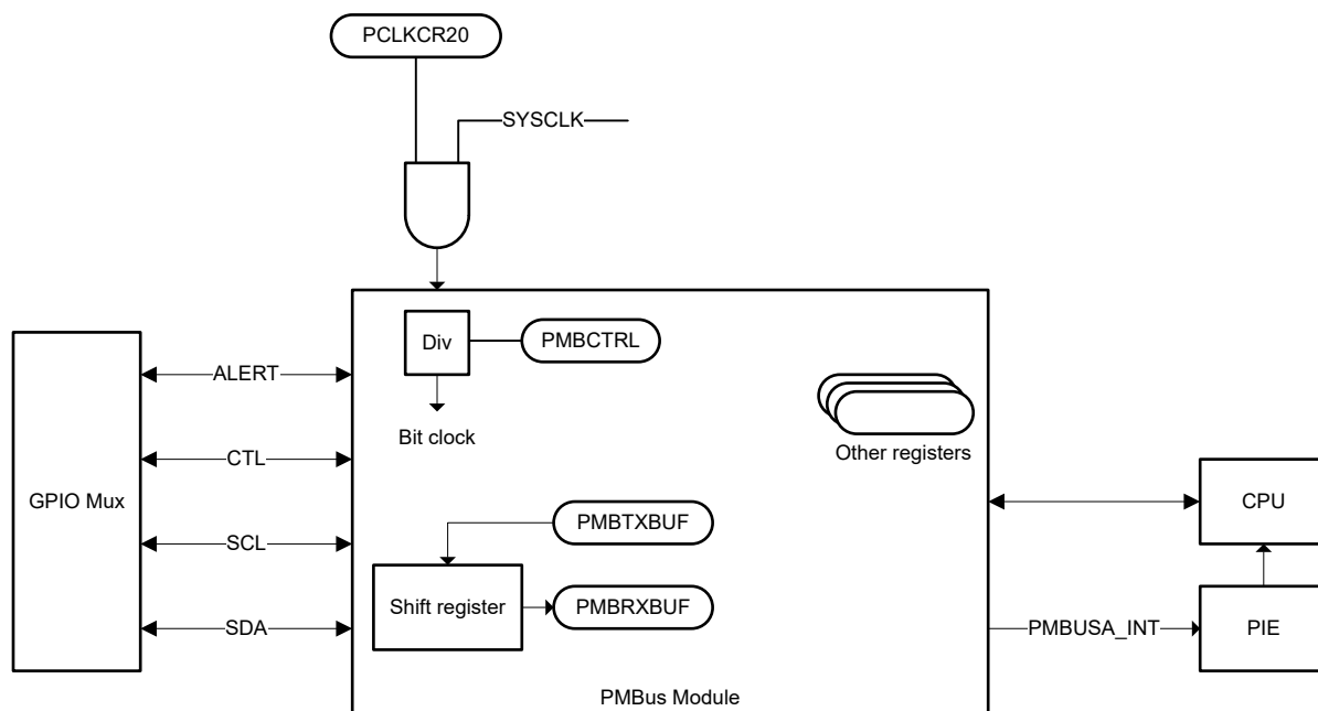
图 6-65. PMBus 方框图
