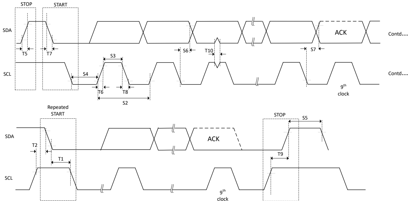
图 6-64. I2C 时序图
