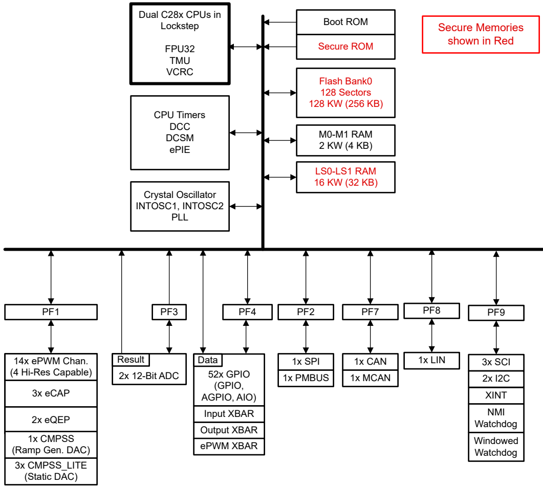
图 7-1. 功能方框图
