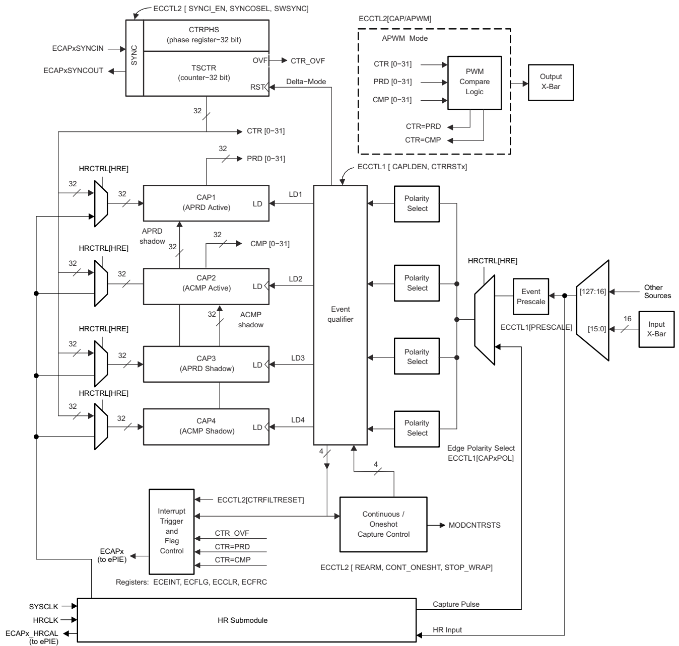
图 6-58. eCAP 方框图
