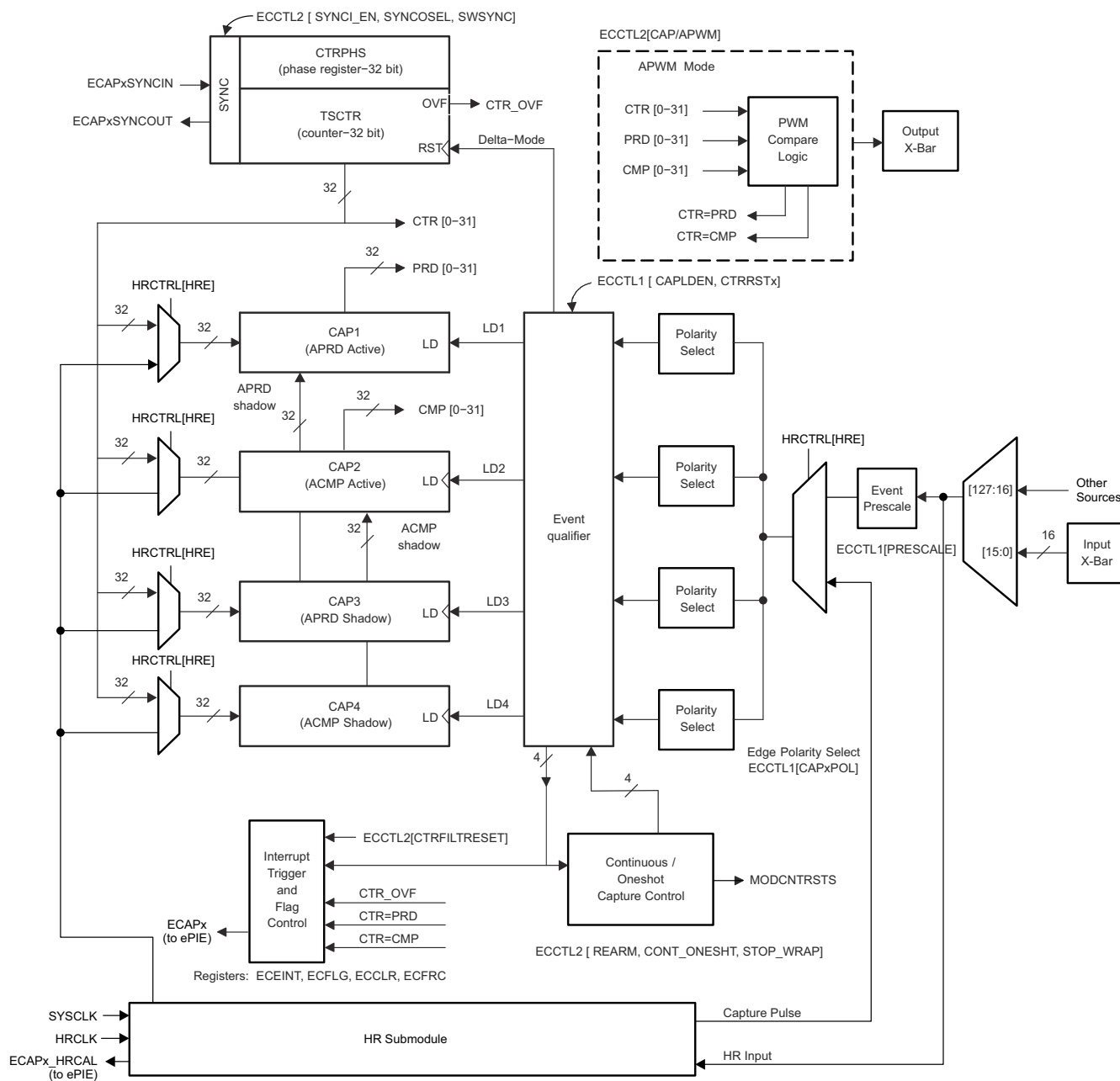
图 6-62. eCAP 方框图
