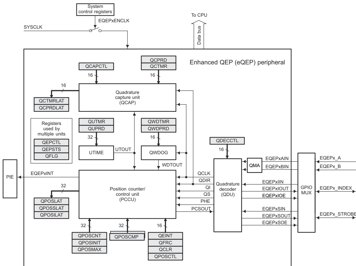
图 6-64. eQEP 方框图
