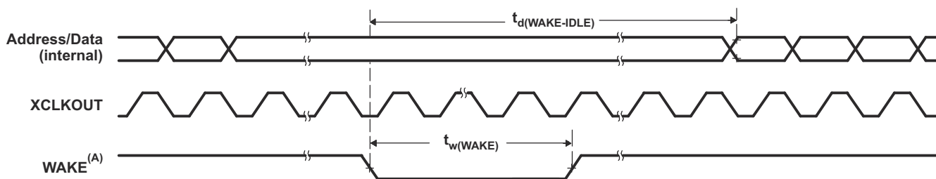
图 6-34. 空闲进入和退出时序图
