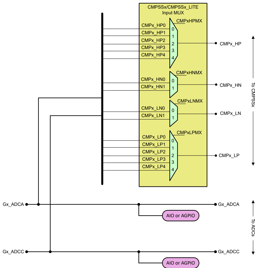
图 6-38. 模拟组连接
