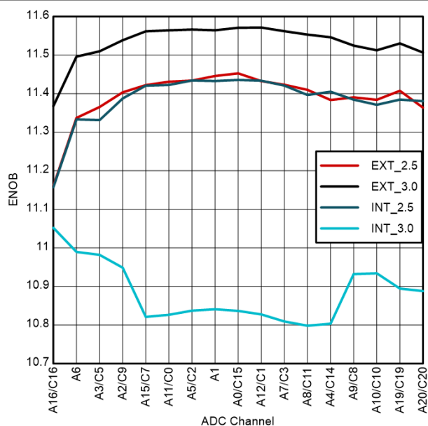
图 6-43. 48 引脚 RGZ VQFN 的每通道 ENOB
