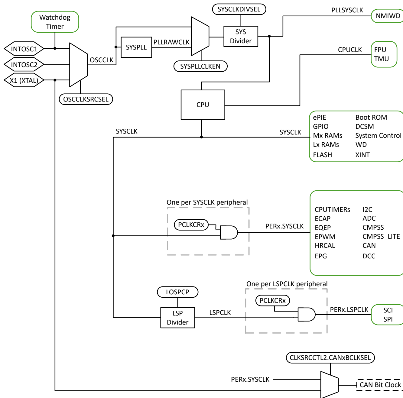
图 6-12. 计时系统
