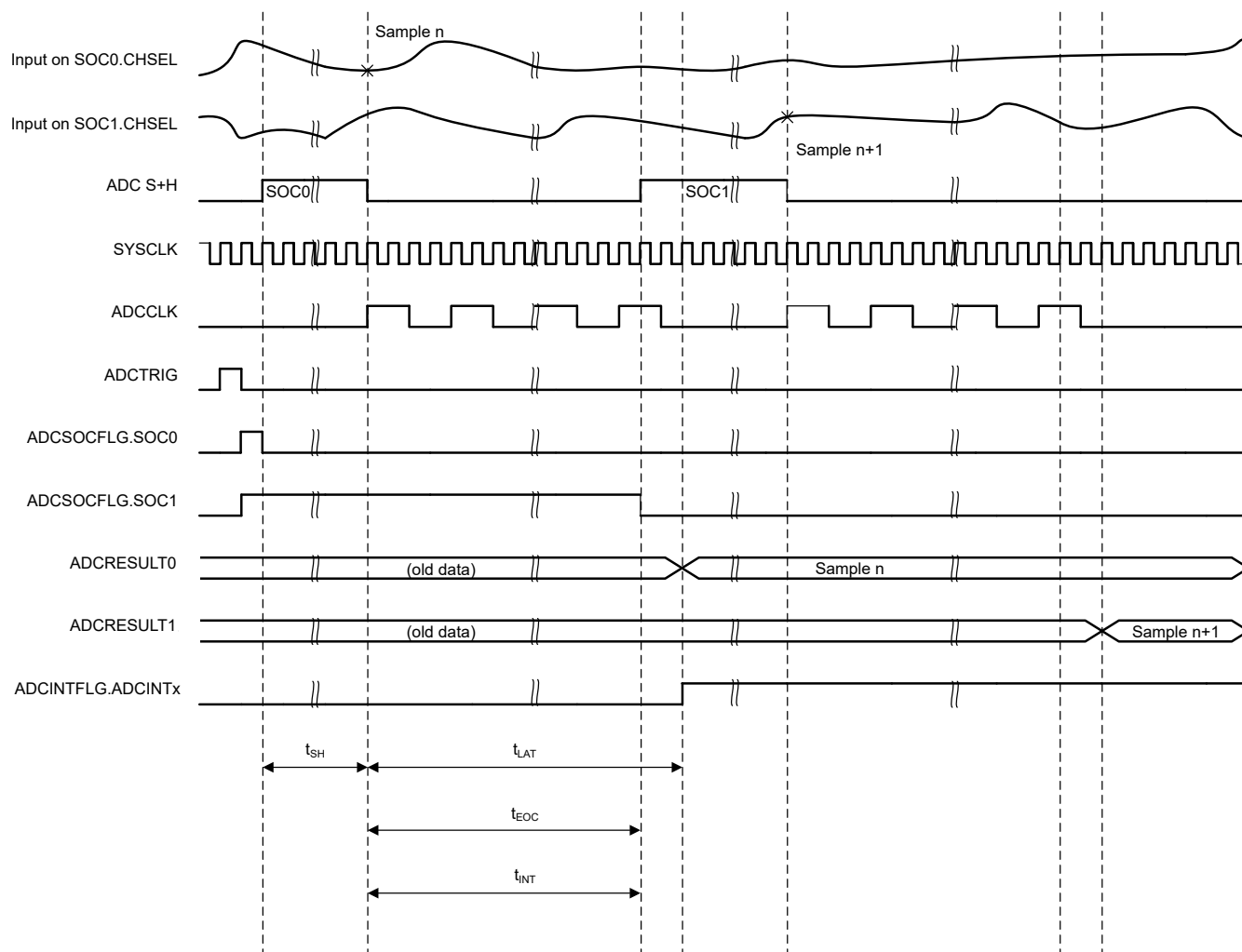
图 6-46. ADC 时序
