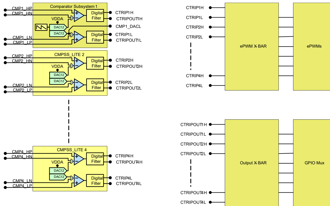
图 6-47. CMPSS 连接
