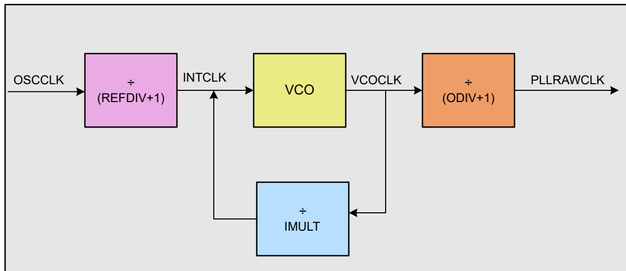
图 6-13. 系统 PLL
