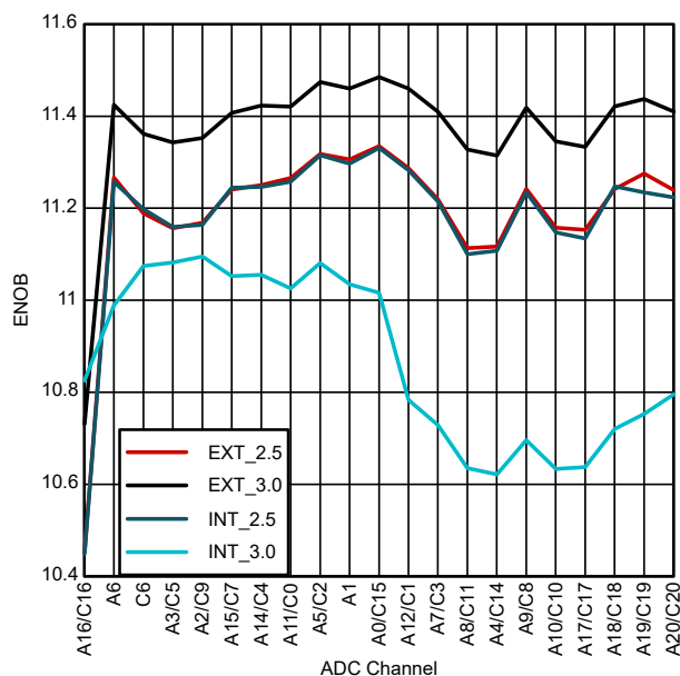
图 6-41. 64 引脚 PM LQFP 的每通道 ENOB
