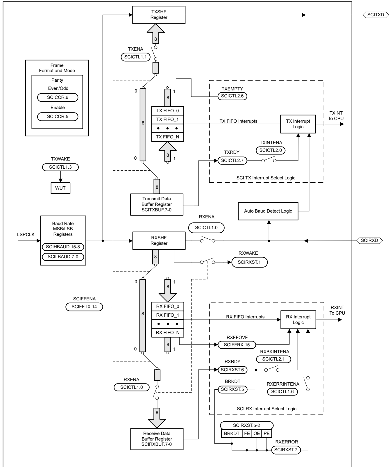
图 6-68. SCI 方框图
