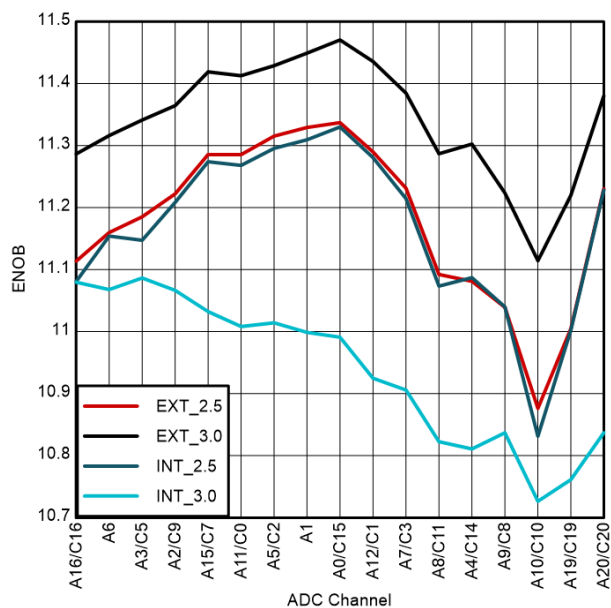
图 6-42. 48 引脚 PT LQFP 的每通道 ENOB
