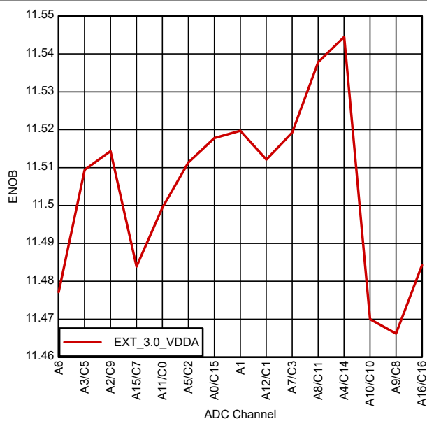
图 6-44. 32 引脚 RHB VQFN 的每通道 ENOB
