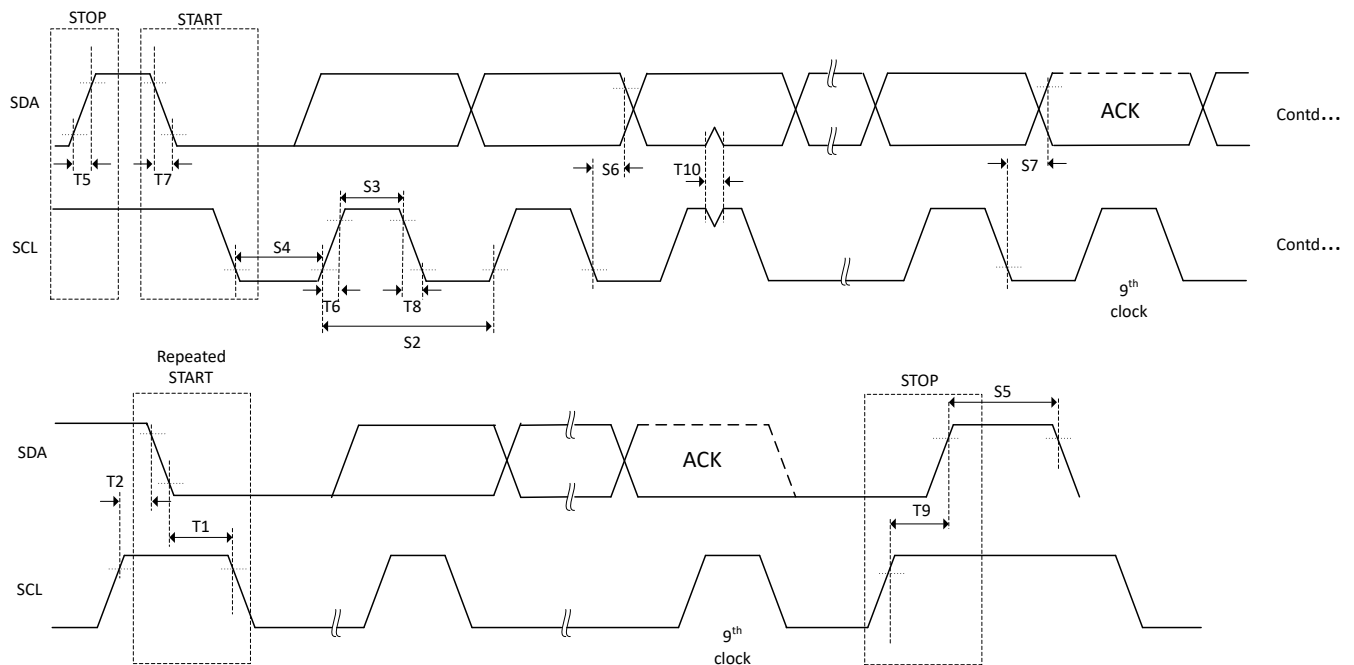
图 6-67. I2C 时序图
