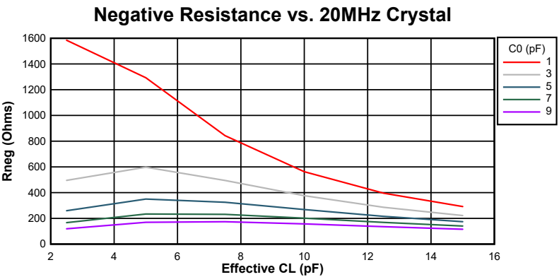
图 6-20. 20MHz 时的负电阻变化
