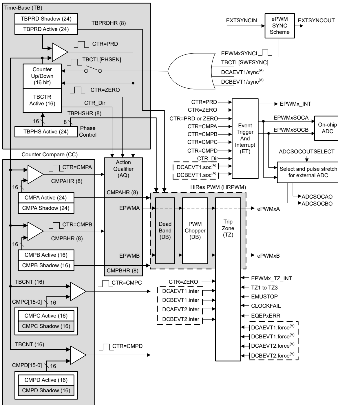
图 6-57. ePWM 子模块和关键内部信号互连
