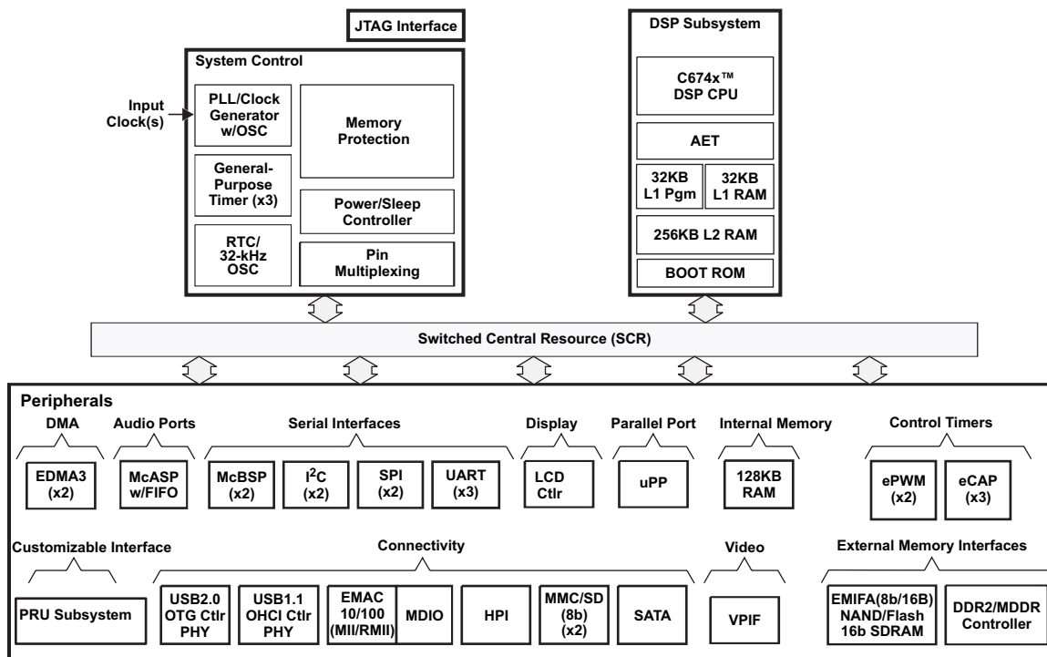
图 1-1. 功能方框图
