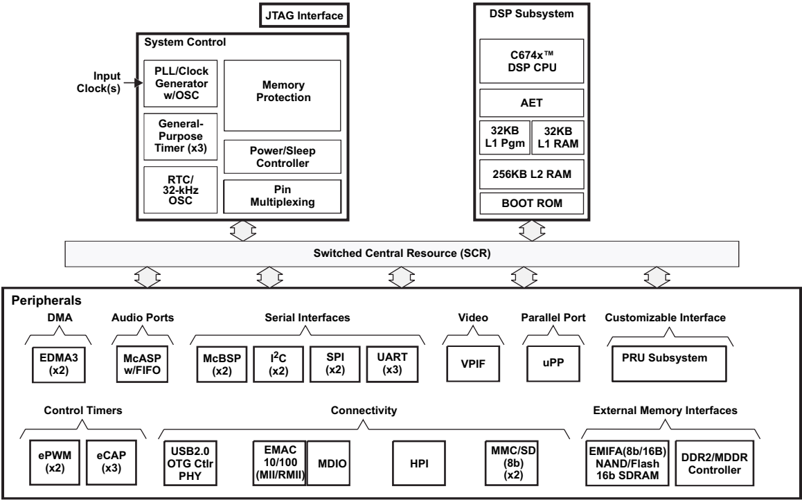
图 1-1. 功能方框图
