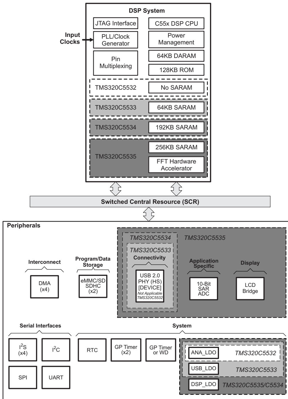
图 1-1. 功能方框图
